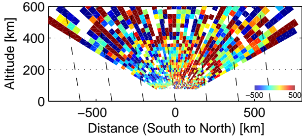
Vi, 83658–83906 UT, 12/3, 2005
