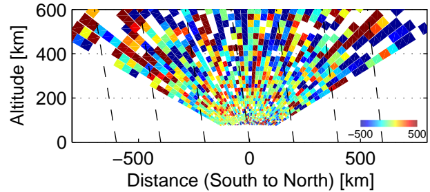
Vi, 74754–75002 UT, 12/3, 2005
