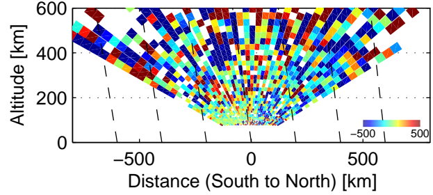
Vi, 73922–74130 UT, 12/3, 2005
