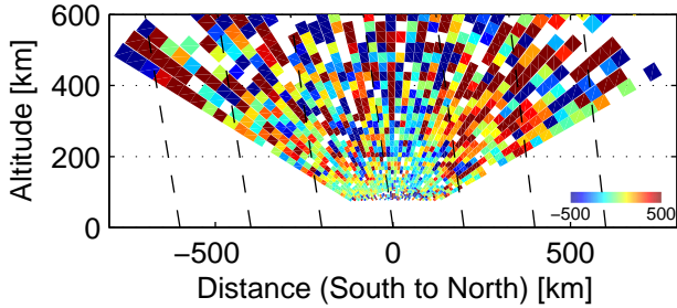
Vi, 83242–83450 UT, 12/3, 2005
