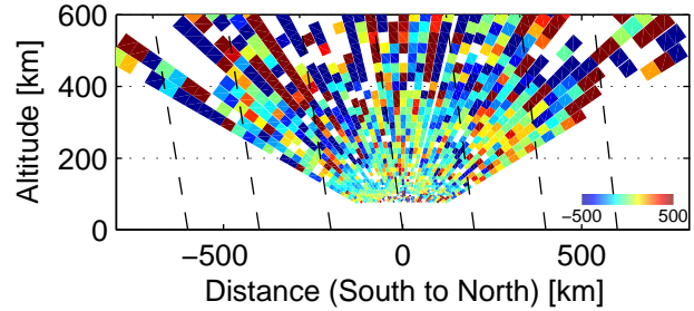
Vi, 82618–82826 UT, 12/3, 2005
