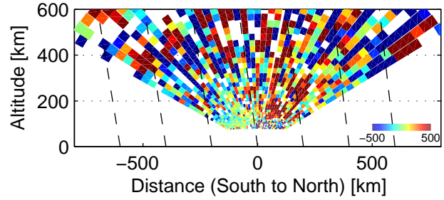
Vi, 83906–84114 UT, 12/3, 2005
