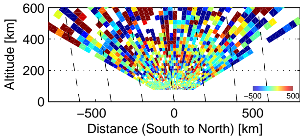
Vi, 94341–94549 UT, 12/4, 2005
