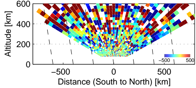
Vi, 93717–93925 UT, 12/4, 2005
