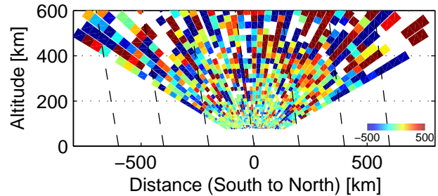
Vi, 95005–95213 UT, 12/4, 2005
