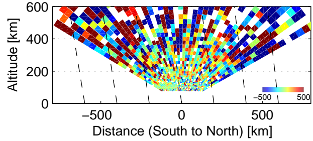
Vi, 93301–93509 UT, 12/4, 2005
