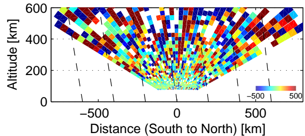
Vi, 94549–94757 UT, 12/4, 2005
