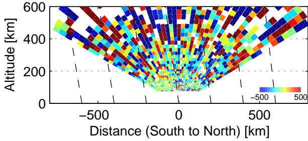
Vi, 93053–93301 UT, 12/4, 2005
