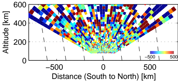
Vi, 94757–95005 UT, 12/4, 2005
