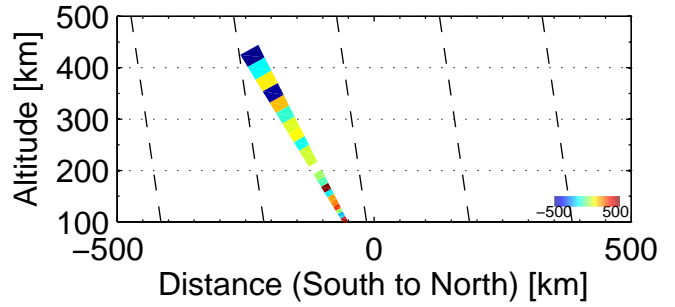
Vi, 204 – 450 UT, 20110111
