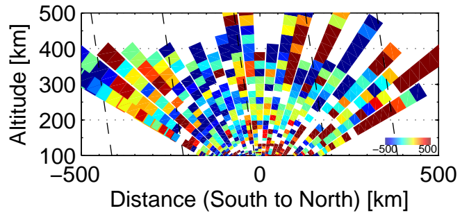
Vi, 730 – 1010 UT, 20110111
