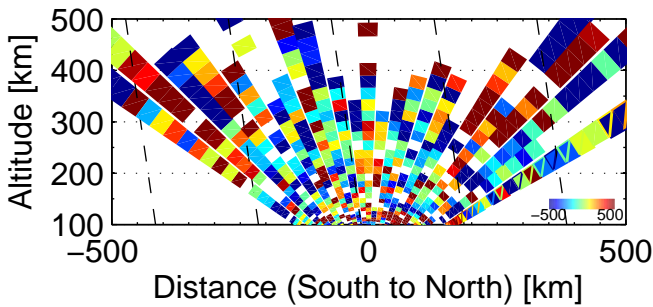
Vi, 1010 – 1250 UT, 20110111
