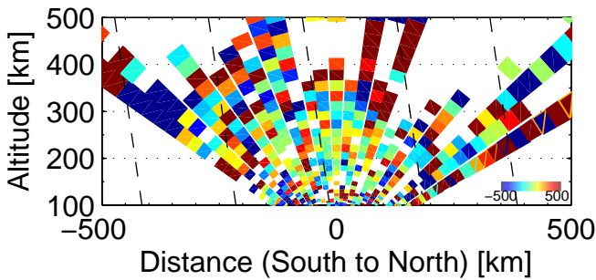
Vi, 1530 – 1804 UT, 20110111
