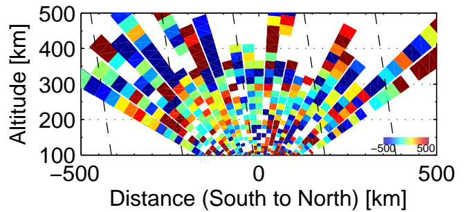
Vi, 1250 – 1530 UT, 20110111
