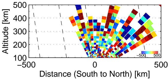
Vi, 450 – 730 UT, 20110111
