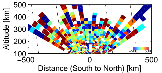
Vi, 1804 – 2050 UT, 20110111
