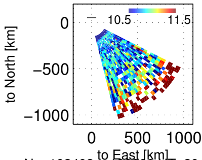
Ne, 102403 – 102800 UT, 20171201
