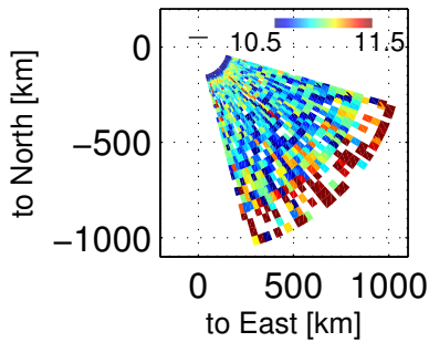
Ne, 72803 – 73200 UT, 20171201
