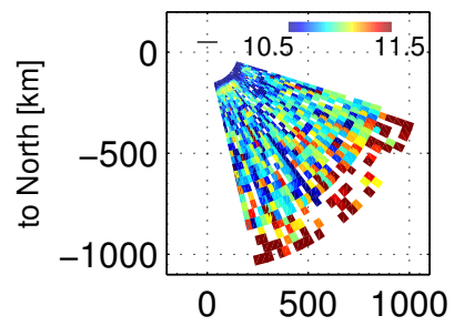
Ne, 102800 – 103203 UT, 20171201
