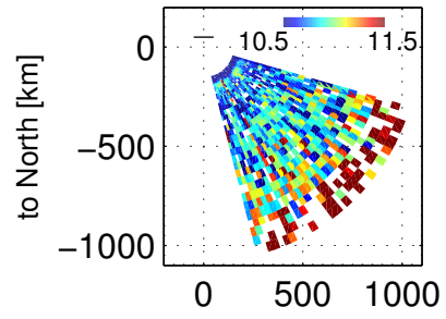
Ne, 100003 – 100400 UT, 20171201
