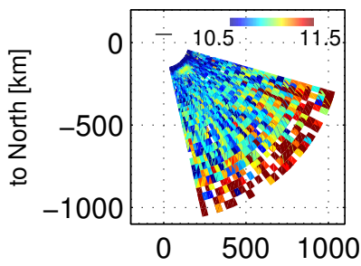
Ne, 102403 – 102800 UT, 20171201
