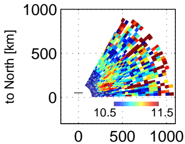
Ne, 104803 – 105200 UT, 20171221
