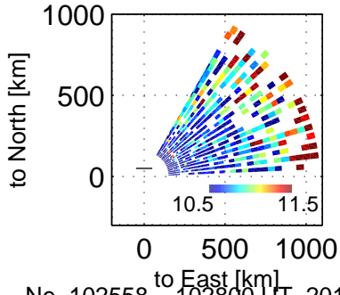
Ne, 102558 – 102800 UT, 20171222
