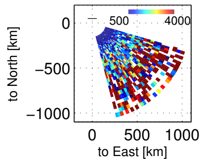
Te, 94403 – 94800 UT, 20171201
