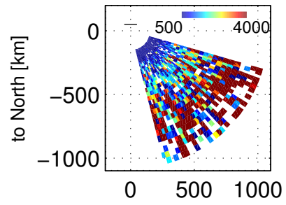
Te, 100757 – 101200 UT, 20171201
