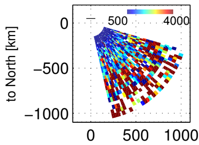
Te, 84803 – 85200 UT, 20171201
