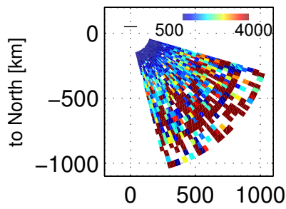
Te, 72803 – 73200 UT, 20171201
