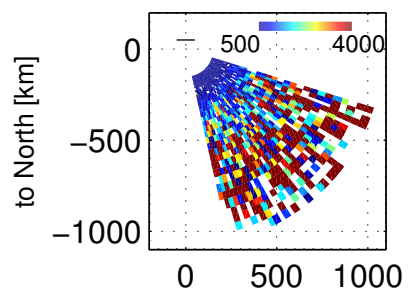
Te, 82000 – 82403 UT, 20171201
