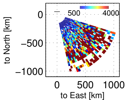
Te, 94000 – 94403 UT, 20171201
