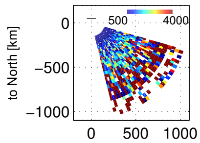
Te, 94403 – 94800 UT, 20171201
