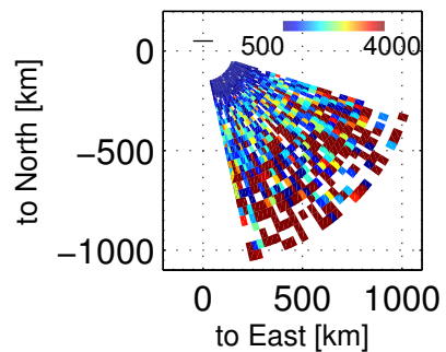
Te, 74000 – 74403 UT, 20171201
