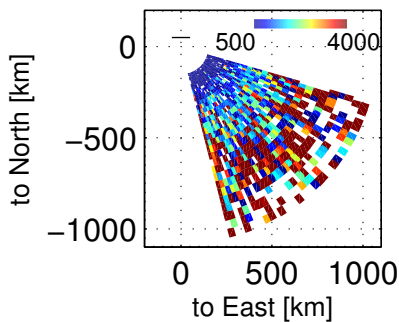
Te, 102403 – 102800 UT, 20171201
