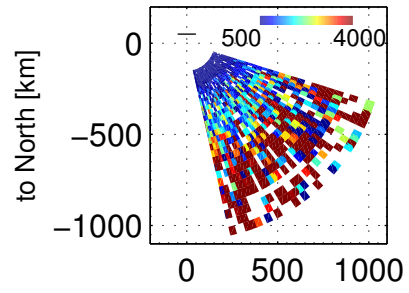
Te, 104400 – 104803 UT, 20171201
