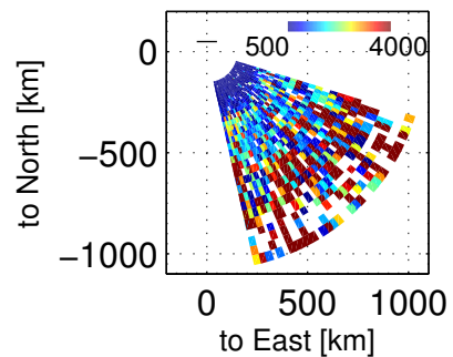
Te, 90000 – 90403 UT, 20171201
