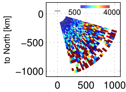
Te, 72003 – 72400 UT, 20171201
