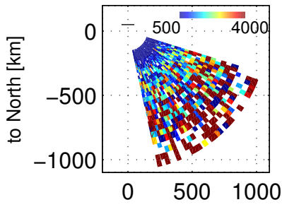
Te, 100400 – 100757 UT, 20171201
