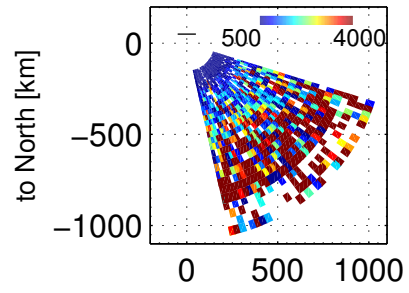
Te, 83600 – 83957 UT, 20171201
