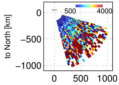
Te, 100003 – 100400 UT, 20171201
