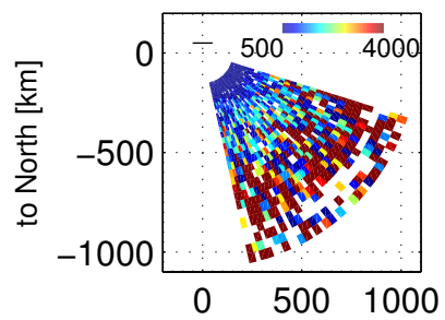
Te, 81200 – 81557 UT, 20171201
