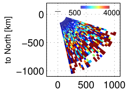
Te, 80400 – 80757 UT, 20171201
