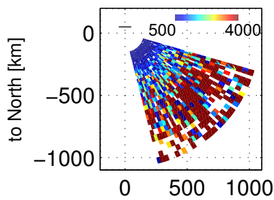
Te, 80757 – 81200 UT, 20171201
