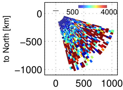
Te, 104803 – 105200 UT, 20171201
