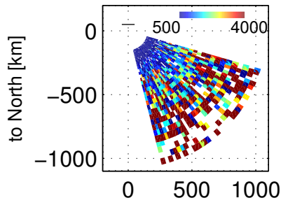
Te, 85603 – 90000 UT, 20171201
