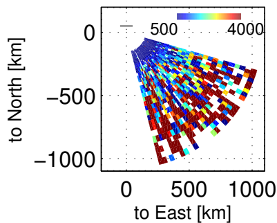
Te, 73603 – 74000 UT, 20171201
