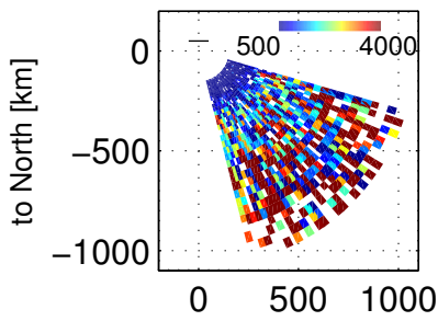
Te, 105603 – 105915 UT, 20171201
