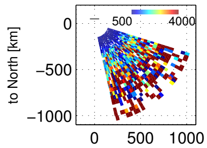
Te, 102000 – 102403 UT, 20171201
