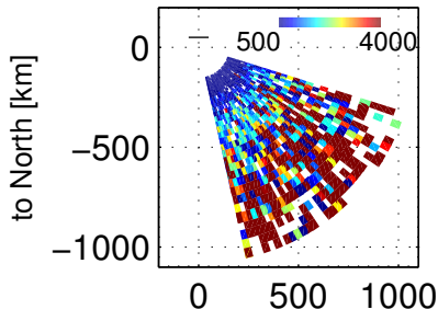
Te, 95600 – 100003 UT, 20171201
