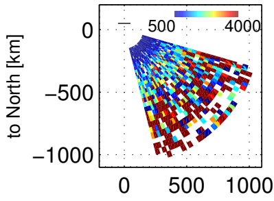
Te, 104003 – 104400 UT, 20171201
