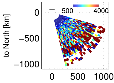
Te, 83203 – 83600 UT, 20171201
