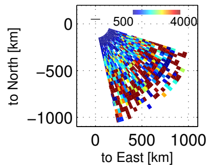
Te, 102800 – 103203 UT, 20171201
