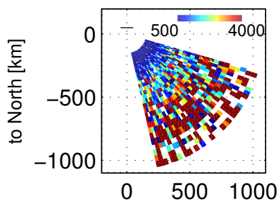
Te, 81557 – 82000 UT, 20171201
