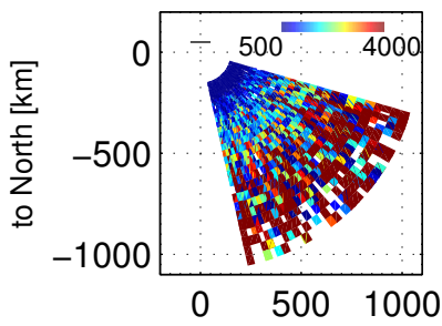
Te, 102403 – 102800 UT, 20171201
