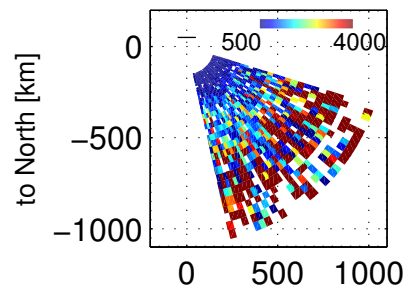
Te, 85200 – 85603 UT, 20171201
