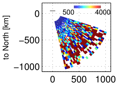
Te, 101200 – 102000 UT, 20171201
