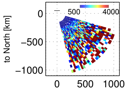
Te, 75203 – 75600 UT, 20171201
