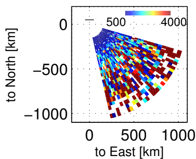
Te, 81557 – 82000 UT, 20171201
