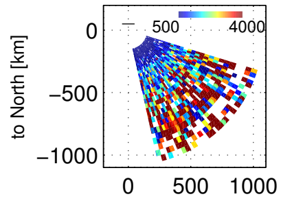
Te, 105200 – 105603 UT, 20171201
