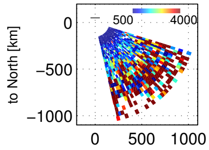
Te, 72400 – 72803 UT, 20171201
