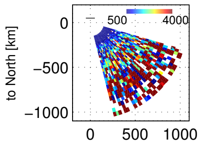
Te, 80003 – 80400 UT, 20171201
