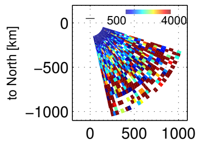
Te, 74000 – 74403 UT, 20171201
