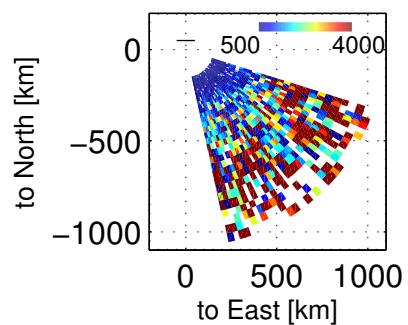
Te, 82000 – 82403 UT, 20171201
