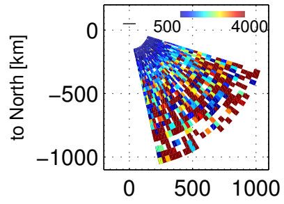
Te, 75600 – 80003 UT, 20171201
