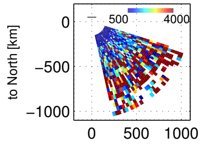
Te, 102800 – 103203 UT, 20171201
