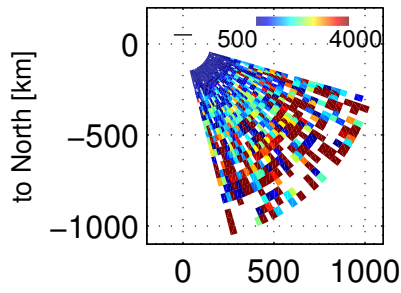
Te, 83957 – 84400 UT, 20171201
