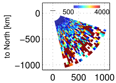
Te, 73200 – 73603 UT, 20171201
