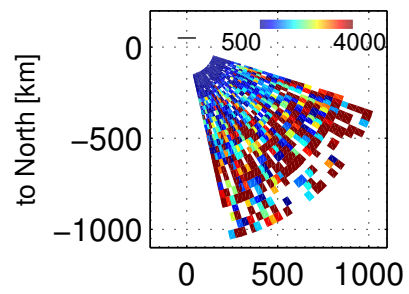
Te, 102800 – 103203 UT, 20171201
