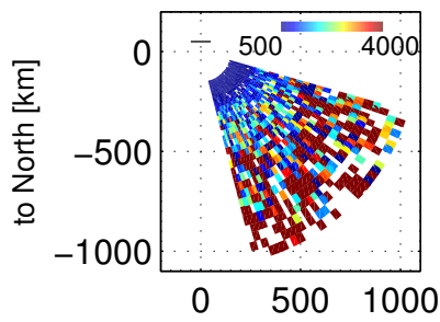
Te, 73603 – 74000 UT, 20171201
