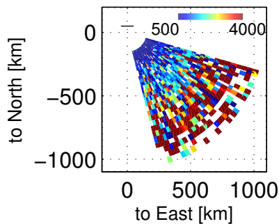
Te, 85603 – 90000 UT, 20171201
