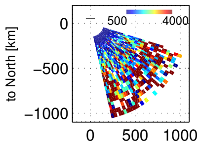
Te, 94000 – 94403 UT, 20171201
