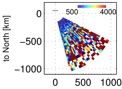
Te, 102403 – 102800 UT, 20171201
