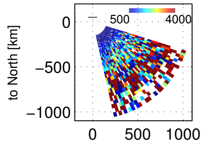
Te, 84400 – 84803 UT, 20171201
