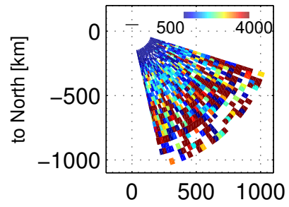
Te, 90000 – 90403 UT, 20171201
