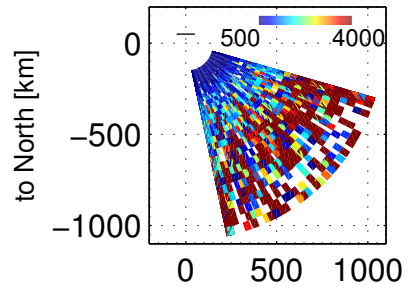
Te, 71600 – 72003 UT, 20171201
