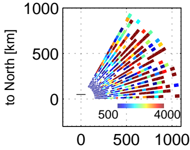
Te, 100602 – 100803 UT, 20171222
