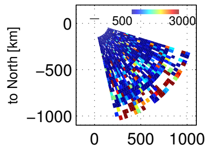
Ti, 105200 – 105603 UT, 20171201
