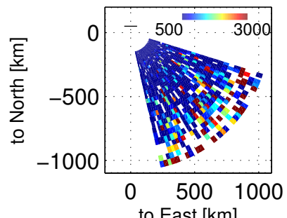
Ti, 73200 – 73603 UT, 20171201
