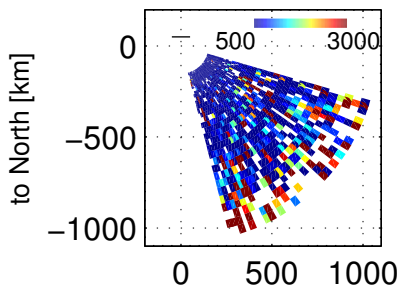
Ti, 104803 – 105200 UT, 20171201
