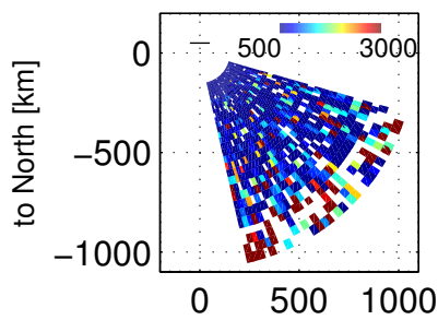
Ti, 84803 – 85200 UT, 20171201
