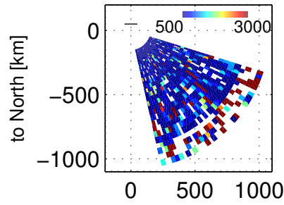
Ti, 104400 – 104803 UT, 20171201
