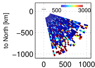
Ti, 102000 – 102403 UT, 20171201
