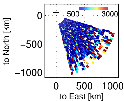
Ti, 102403 – 102800 UT, 20171201
