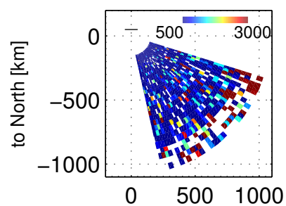
Ti, 90000 – 90403 UT, 20171201
