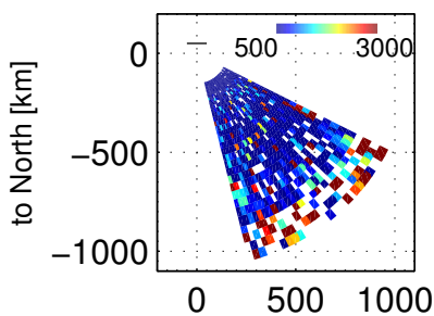
Ti, 102403 – 102800 UT, 20171201
