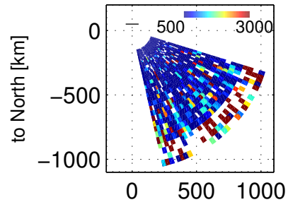
Ti, 83600 – 83957 UT, 20171201
