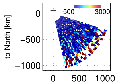
Ti, 84400 – 84803 UT, 20171201
