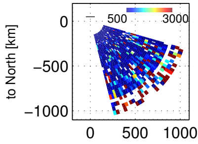
Ti, 83203 – 83600 UT, 20171201
