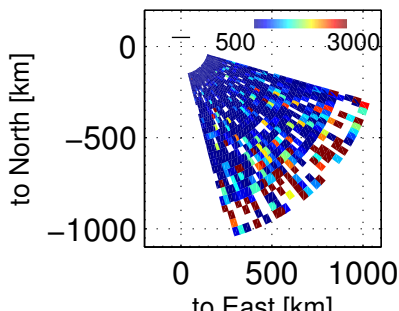
Ti, 72803 – 73200 UT, 20171201
