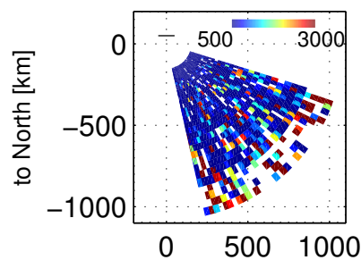
Ti, 102800 – 103203 UT, 20171201
