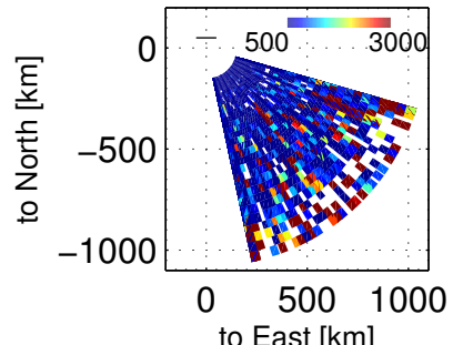
Ti, 71600 – 72003 UT, 20171201
