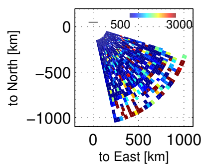
Ti, 90000 – 90403 UT, 20171201
