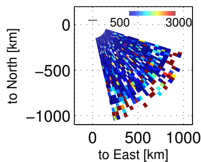
Ti, 102800 – 103203 UT, 20171201
