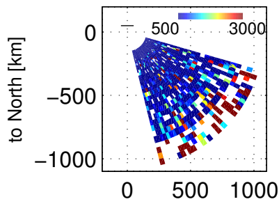
Ti, 83957 – 84400 UT, 20171201
