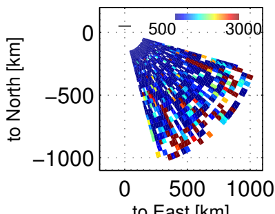
Ti, 73603 – 74000 UT, 20171201
