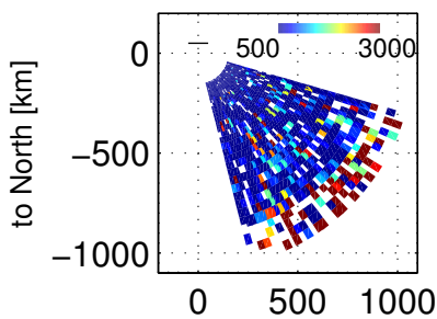
Ti, 105603 – 105915 UT, 20171201
