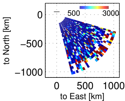
Ti, 73603 – 74000 UT, 20171201
