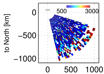
Ti, 85200 – 85603 UT, 20171201
