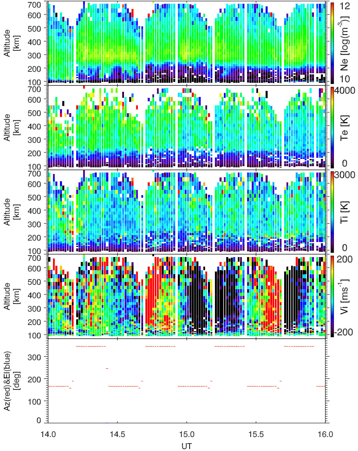
EISCAT 1998-10-21_14_16UT_gup3c_ant@32m.
