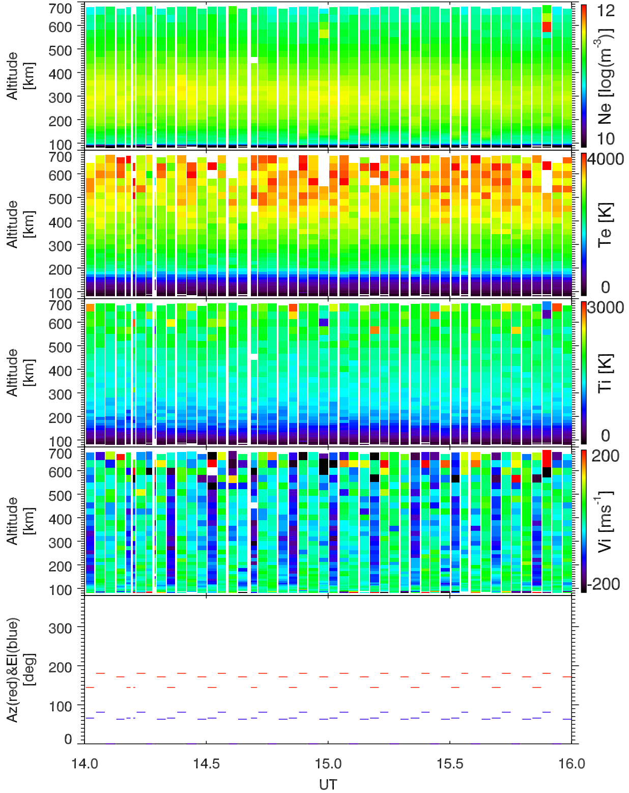
EISCAT 1999-07-01_14_16UT_gup3c_ant@32m.
