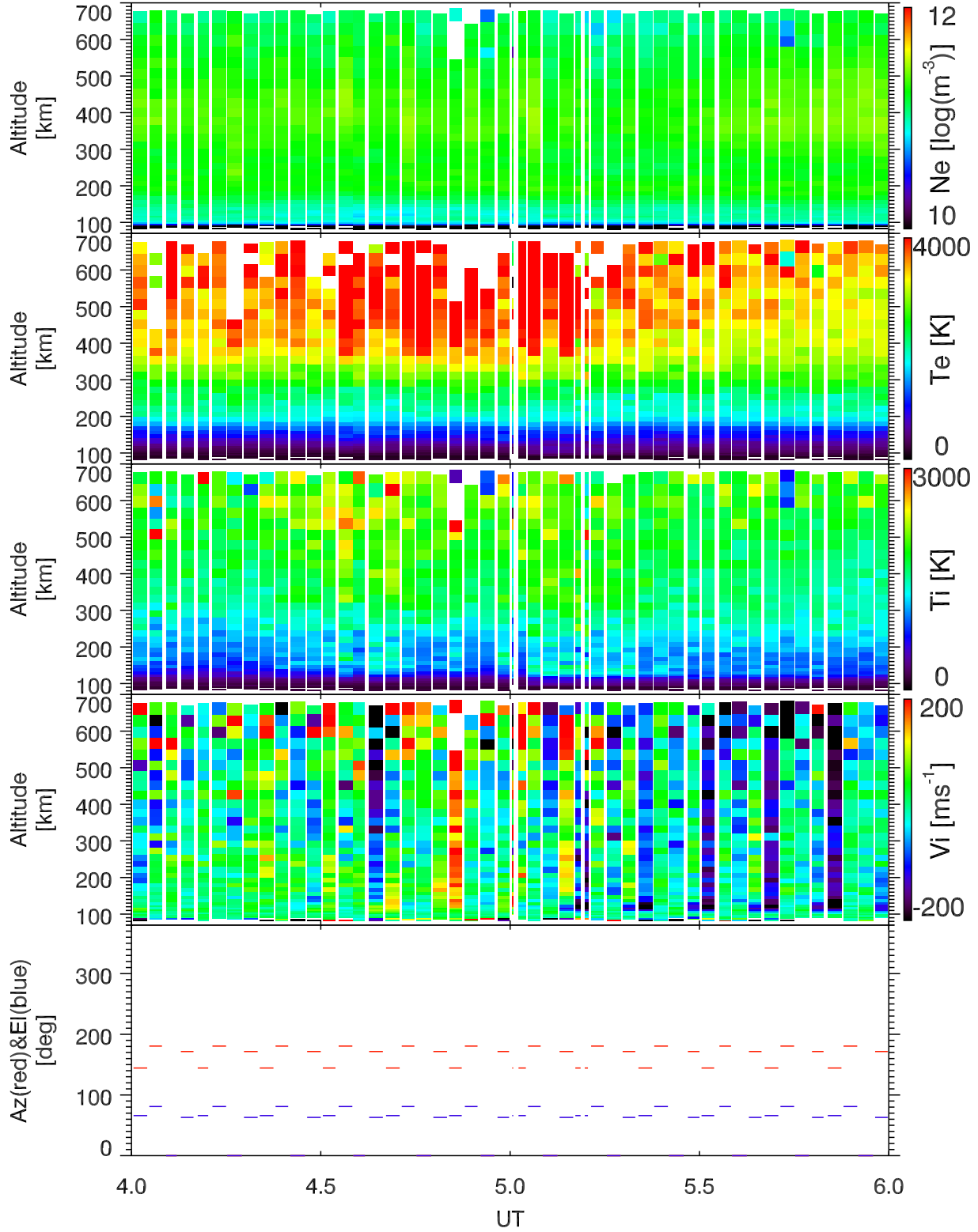
EISCAT 1999-07-02_04_06UT_gup3c_ant@32m.
