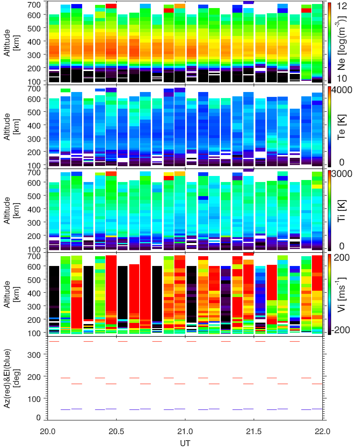
EISCAT 2000-03-15_20_22UT_gup3c_ant@32m.
