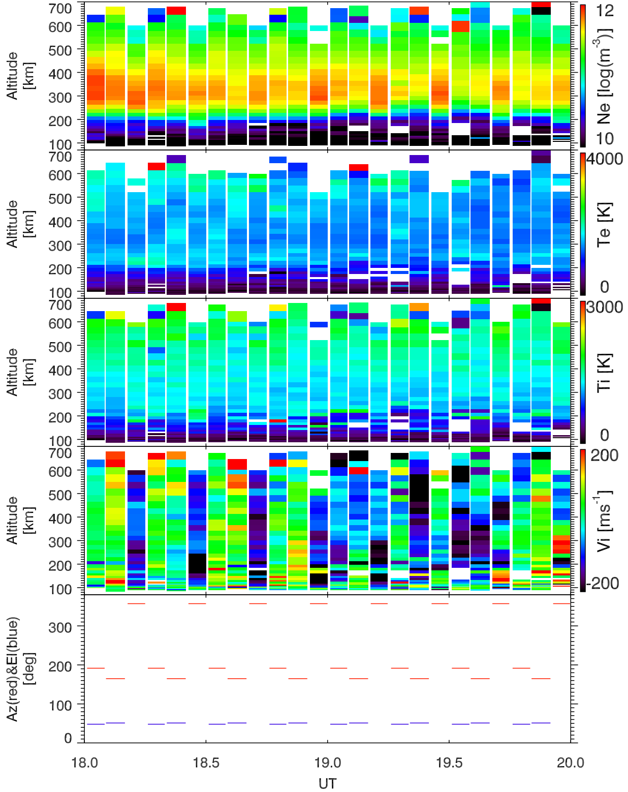
EISCAT 2000-03-16_18_20UT_gup3c_ant@32m.
