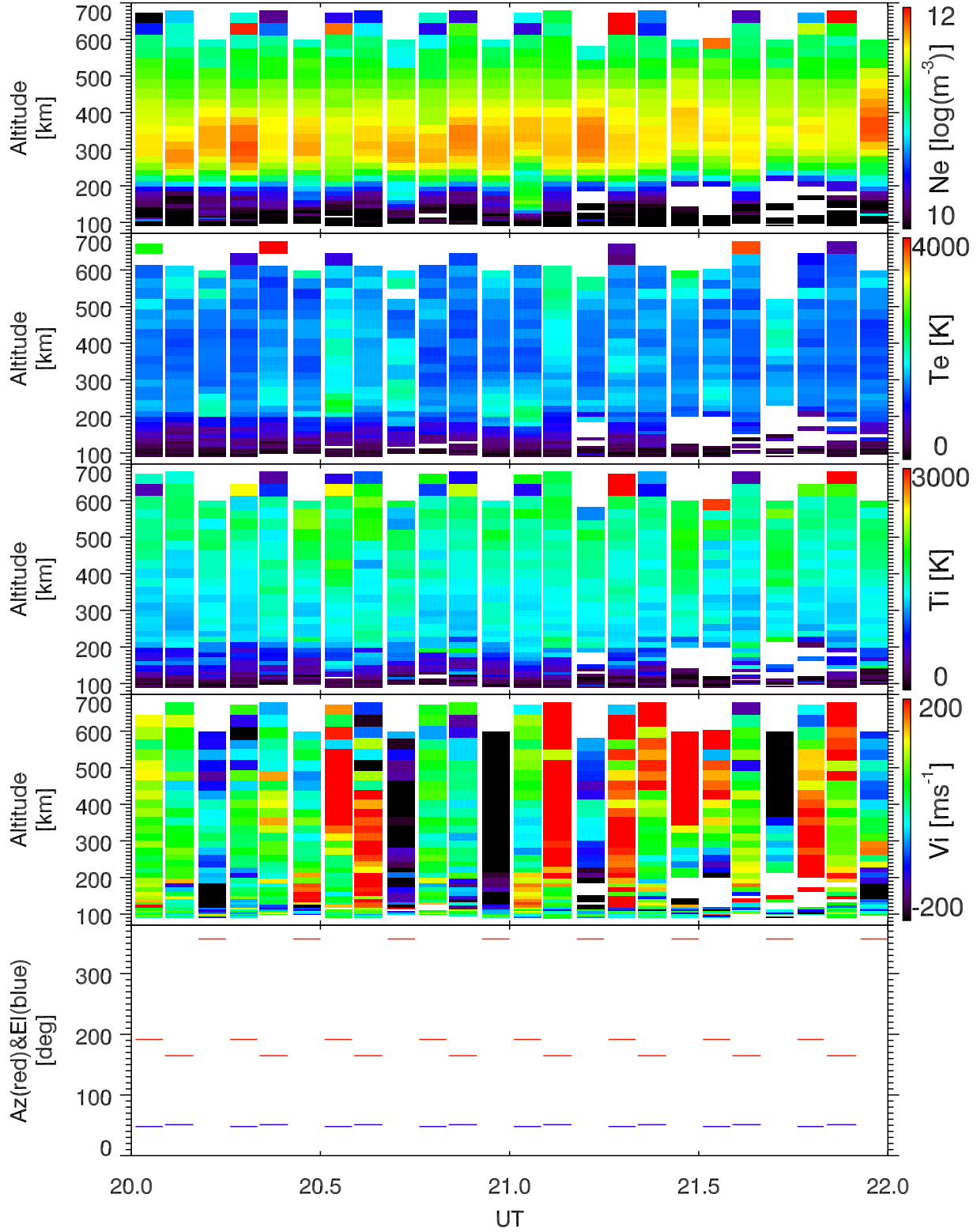
EISCAT 2000-03-16_20_22UT_gup3c_ant@32m.
