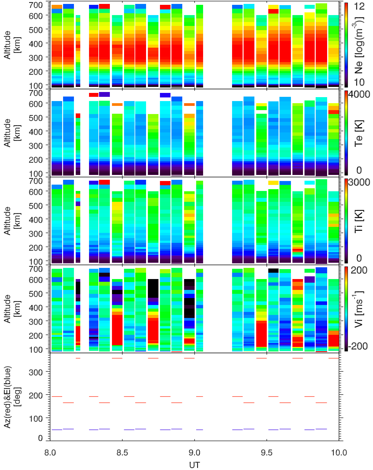
EISCAT 2000-03-17_08_10UT_gup3c_ant@32m.
