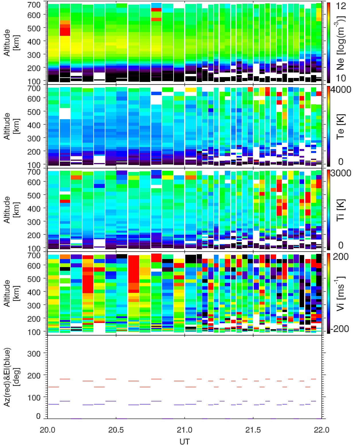
EISCAT 2000-03-17_20_22UT_gup3c_ant@32m.
