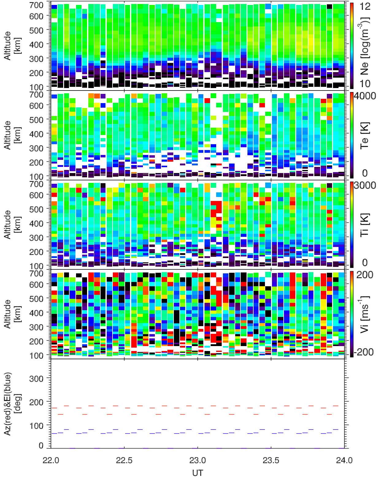
EISCAT 2000-03-17_22_24UT_gup3c_ant@32m.
