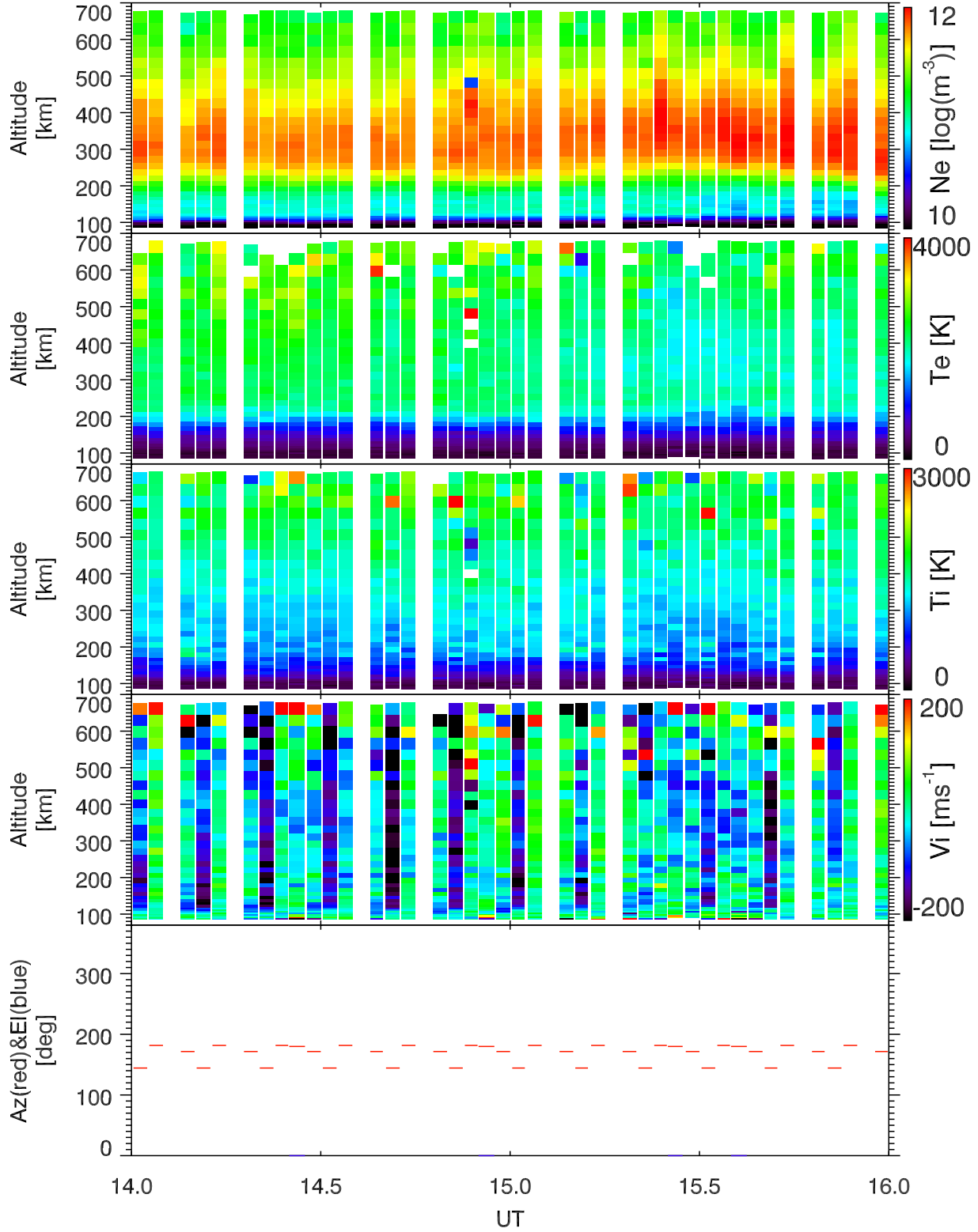
EISCAT 2000-03-18_14_16UT_gup3c_ant@32m.
