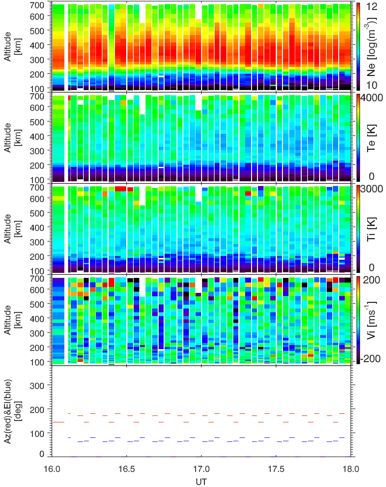
EISCAT 2000-03-18_16_18UT_gup3c_ant@32m.
