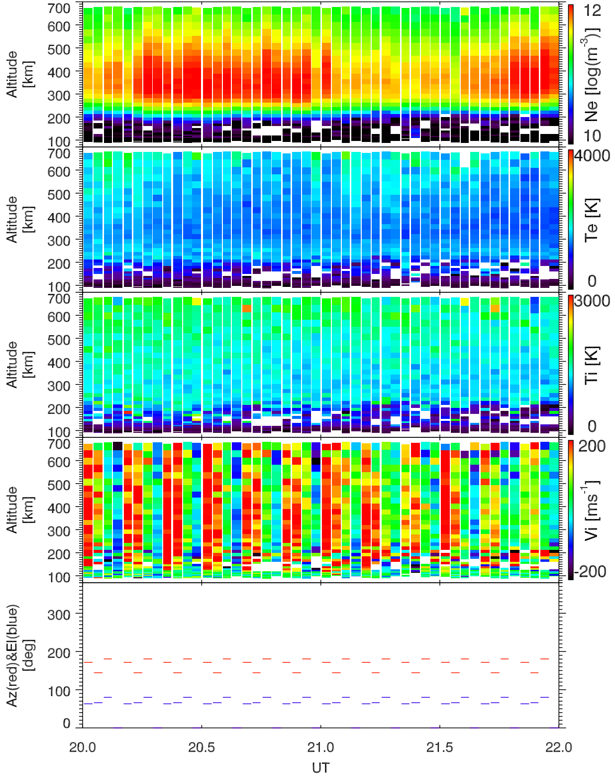
EISCAT 2000-03-18_20_22UT_gup3c_ant@32m.
