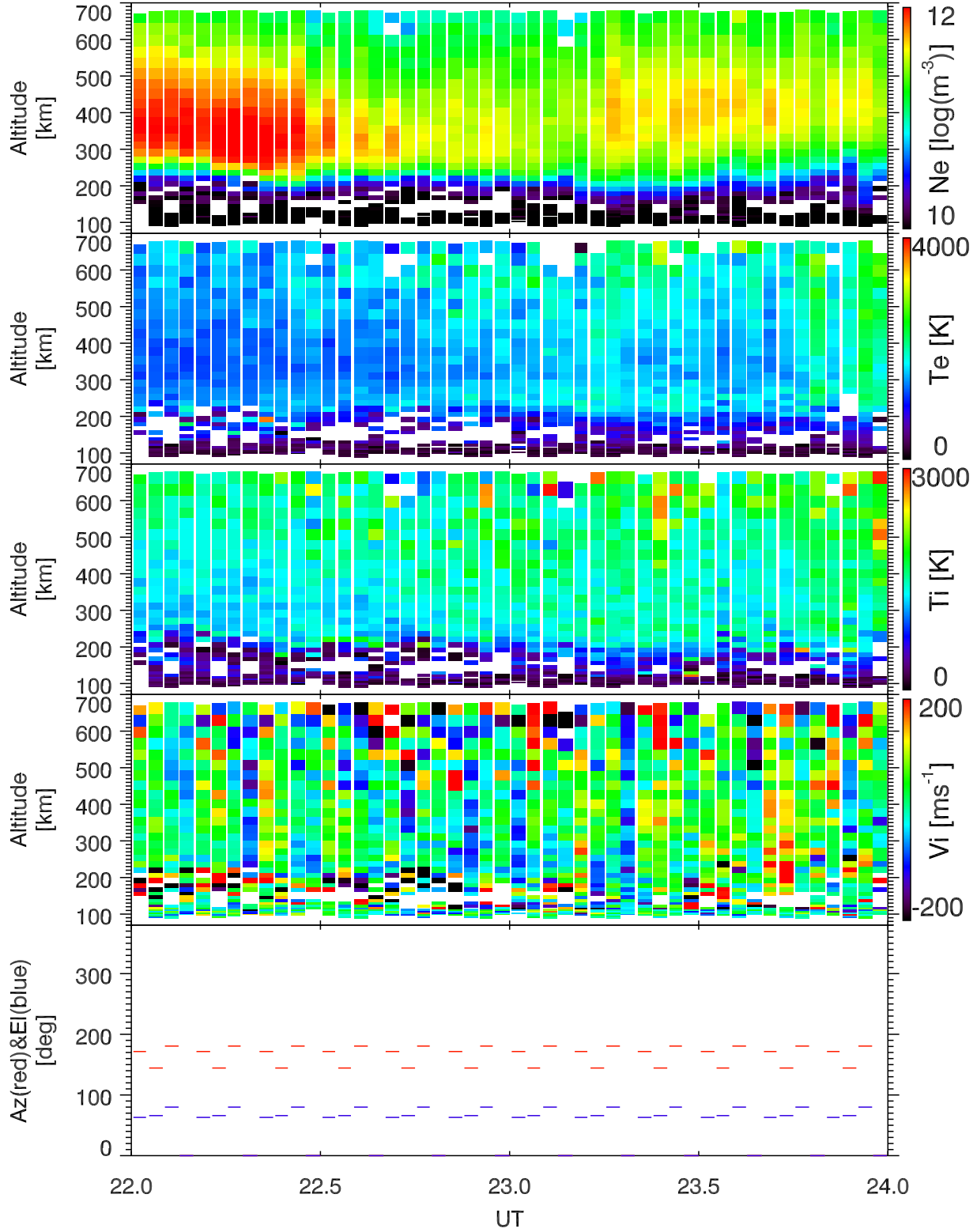
EISCAT 2000-03-18_22_24UT_gup3c_ant@32m.
