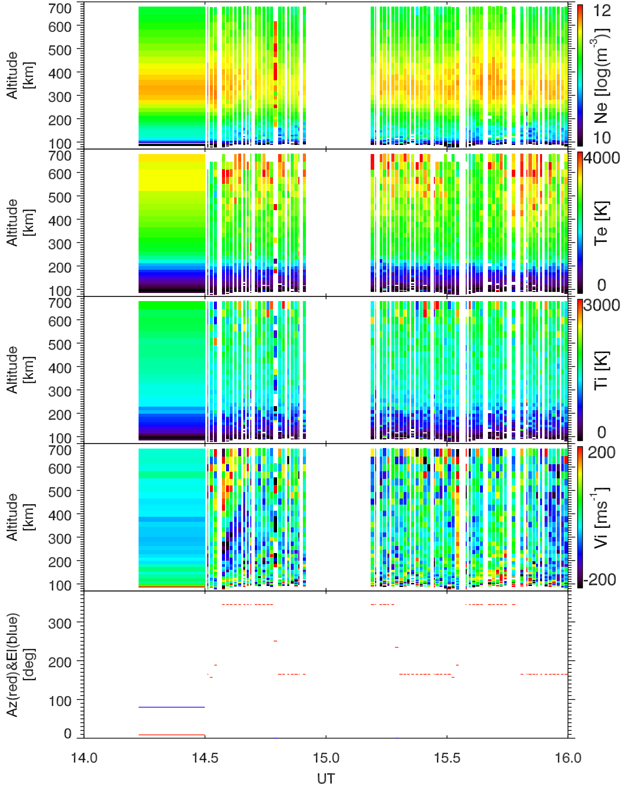
EISCAT 2000-04-12_14_16UT_tau0_ant@32m.
