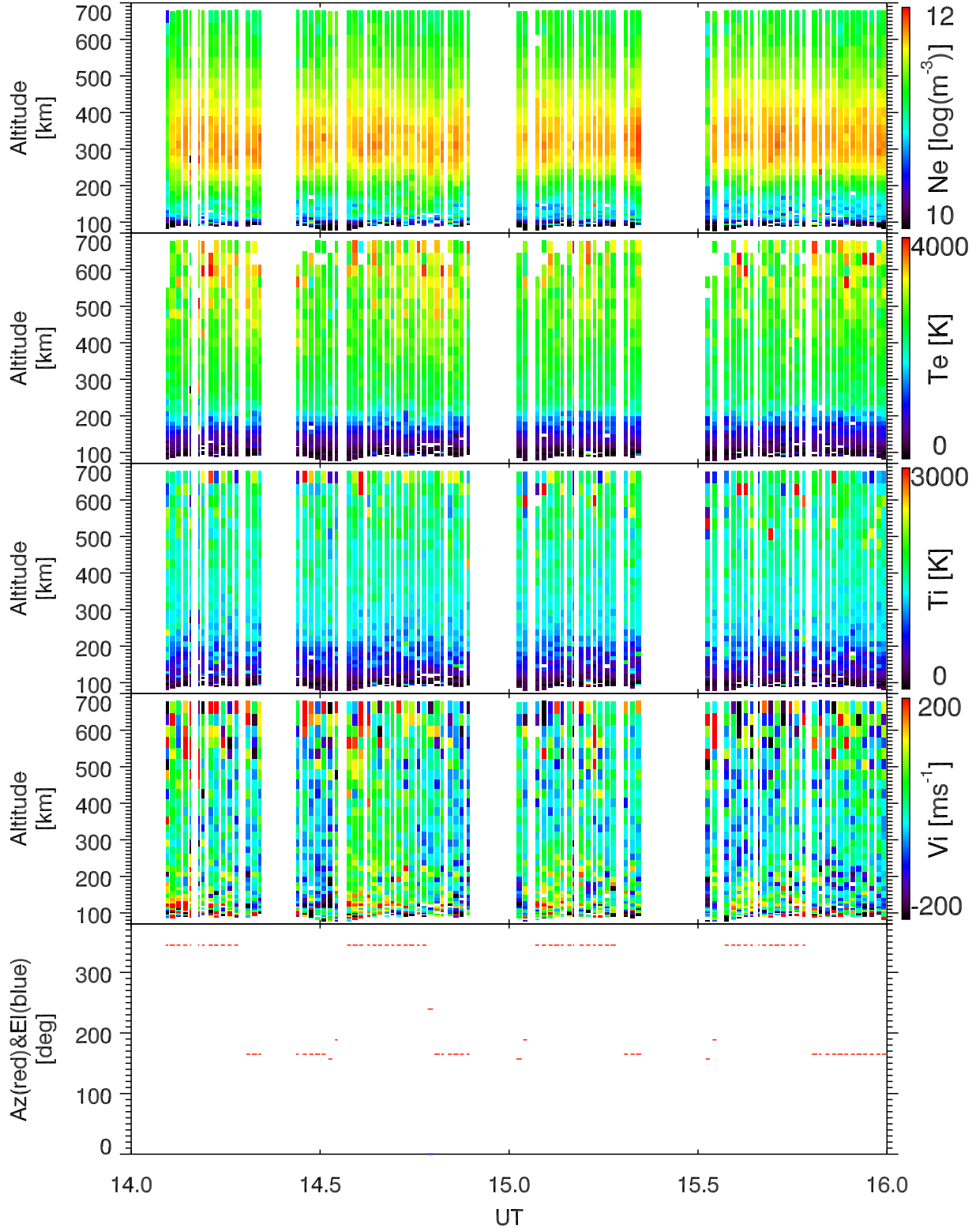
EISCAT 2000-04-13_14_16UT_tau0_ant@32m.
