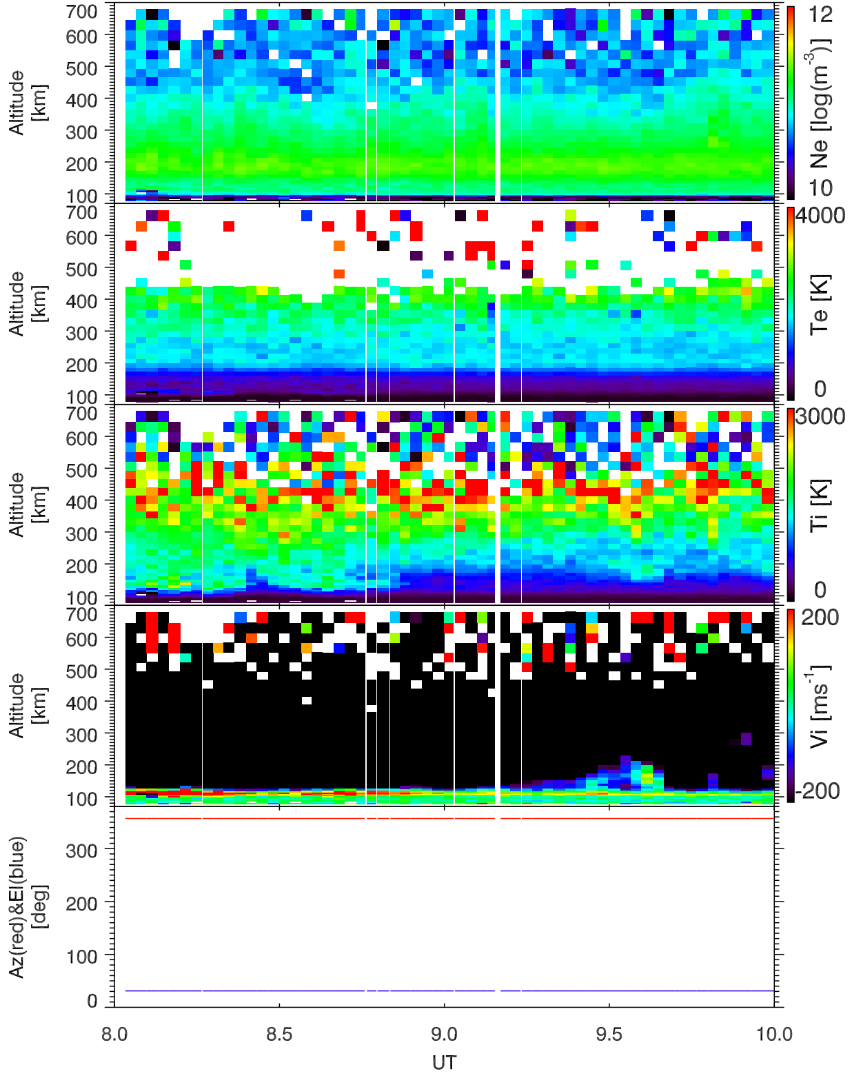
EISCAT 2000-07-16_08_10UT_tau0_120@32m.
