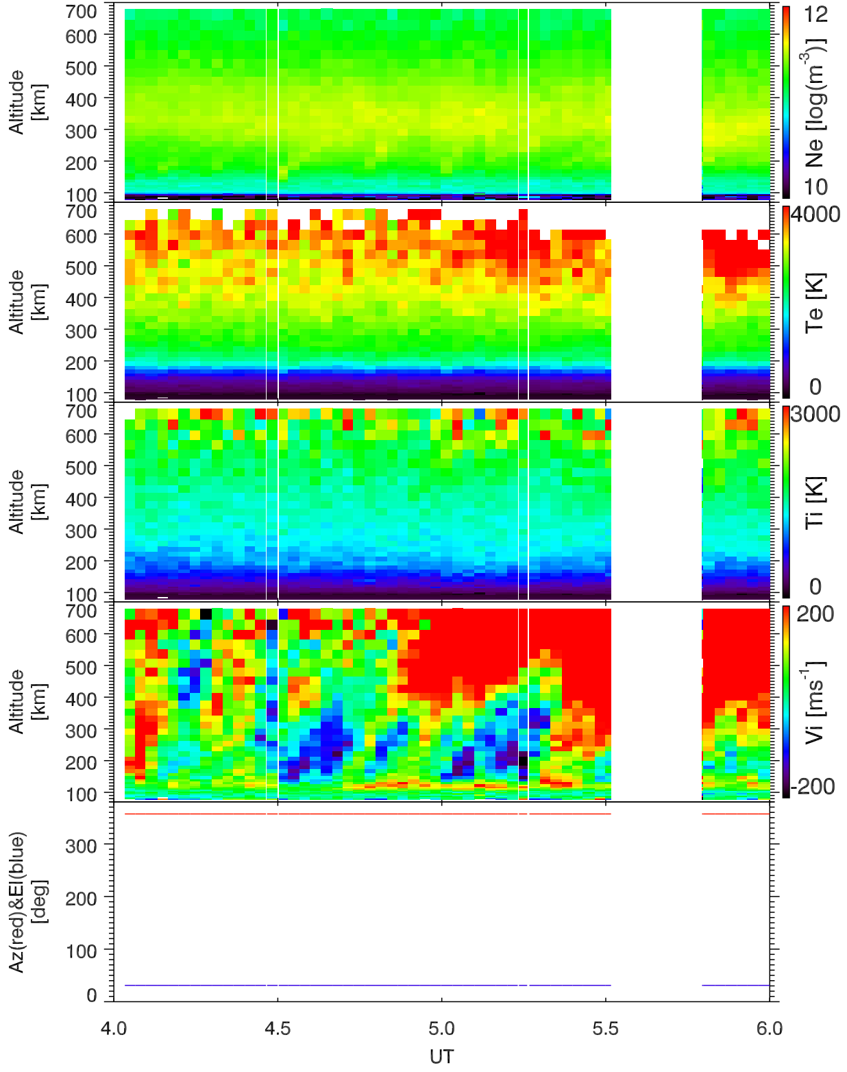
EISCAT 2000-07-17_04_06UT_tau0_120@32m.
