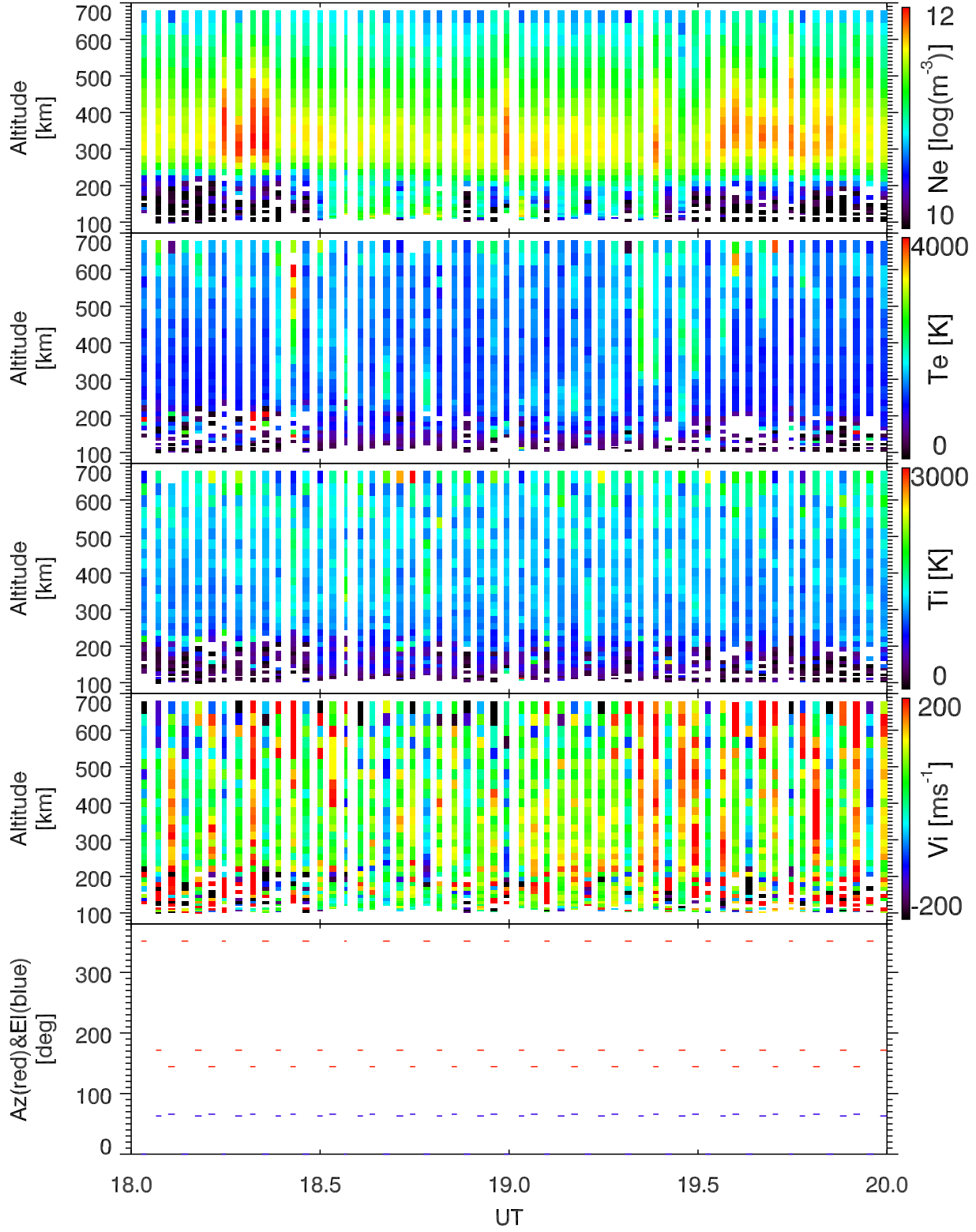
EISCAT 2001-02-17_18_20UT_tau0_ant@32m.
