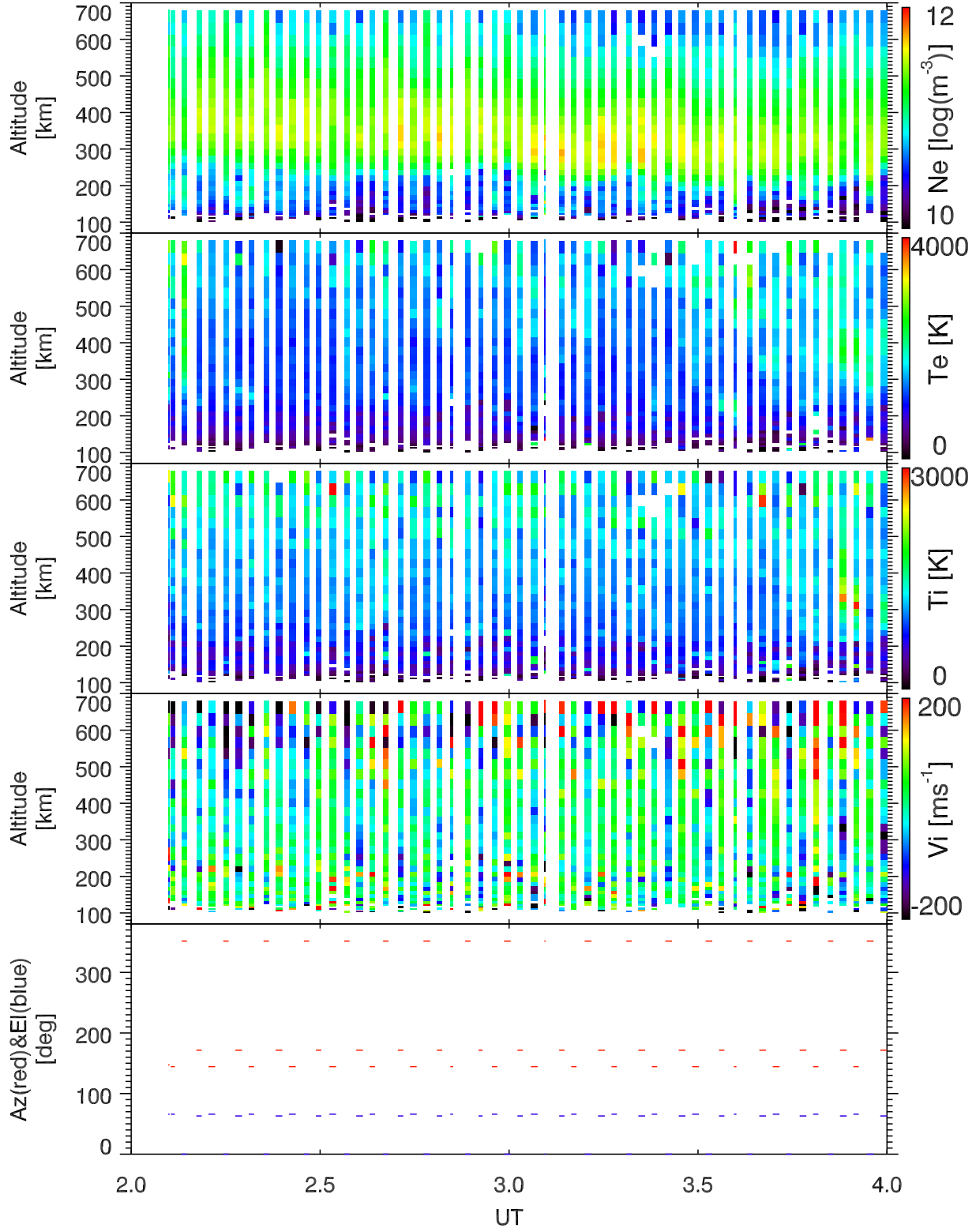
EISCAT 2001-02-18_02_04UT_tau0_ant@32m.
