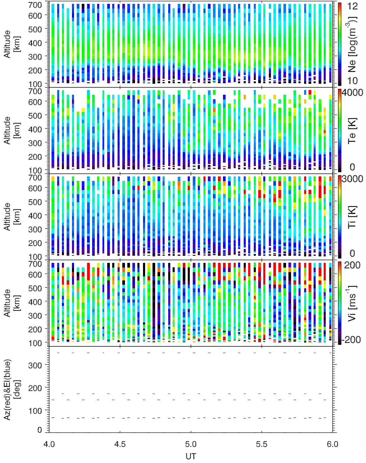
EISCAT 2001-02-19_04_06UT_tau0_ant@32m.
