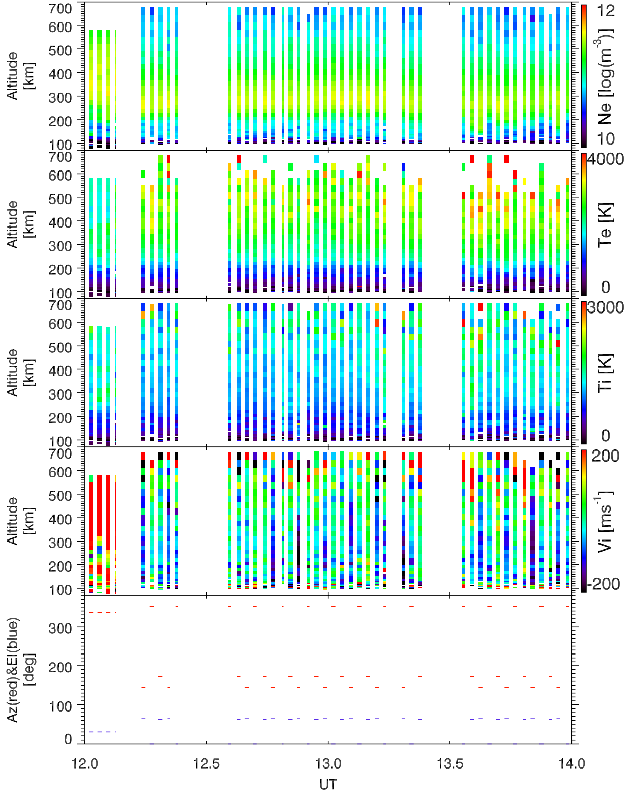
EISCAT 2001-02-19_12_14UT_tau0_ant@32m.
