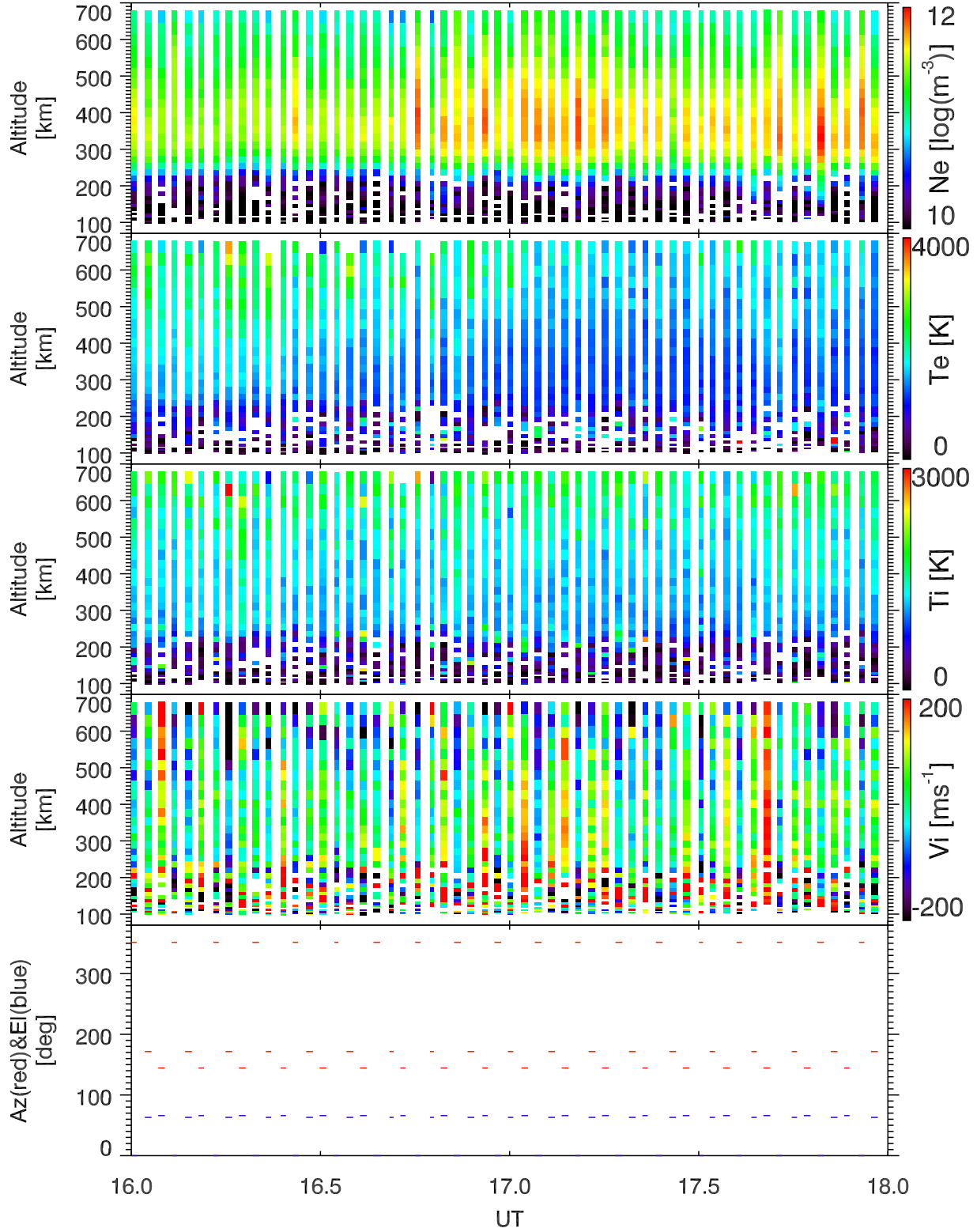
EISCAT 2001-02-19_16_18UT_tau0_ant@32m.
