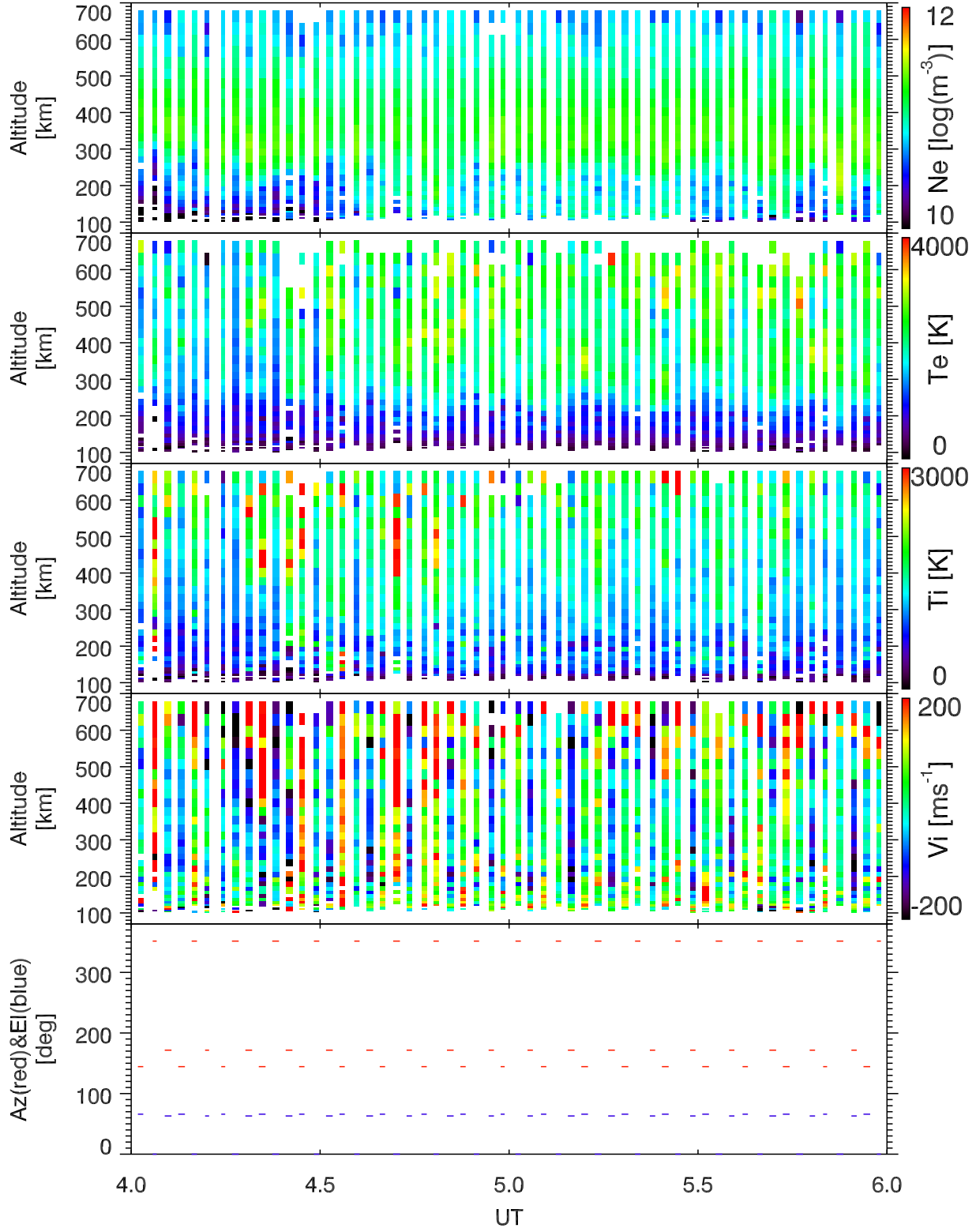
EISCAT 2001-02-20_04_06UT_tau0_ant@32m.
