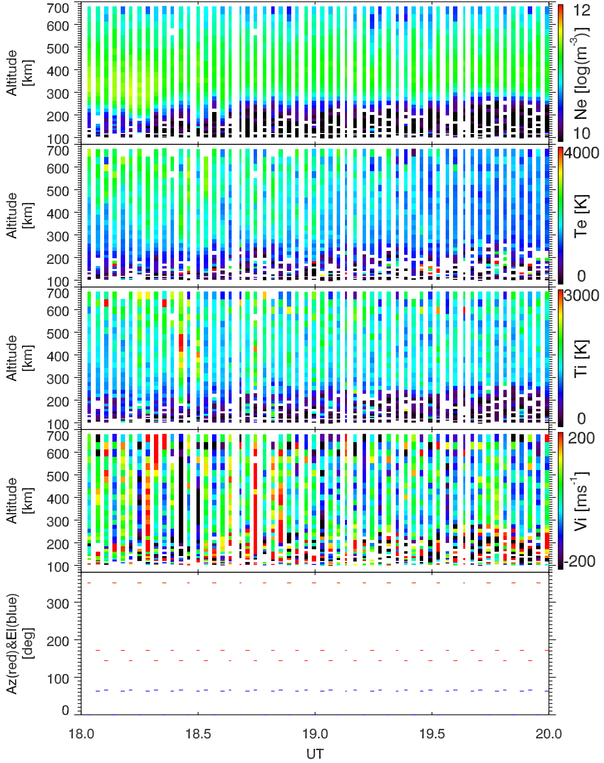
EISCAT 2001-02-20_18_20UT_tau0_ant@32m.
