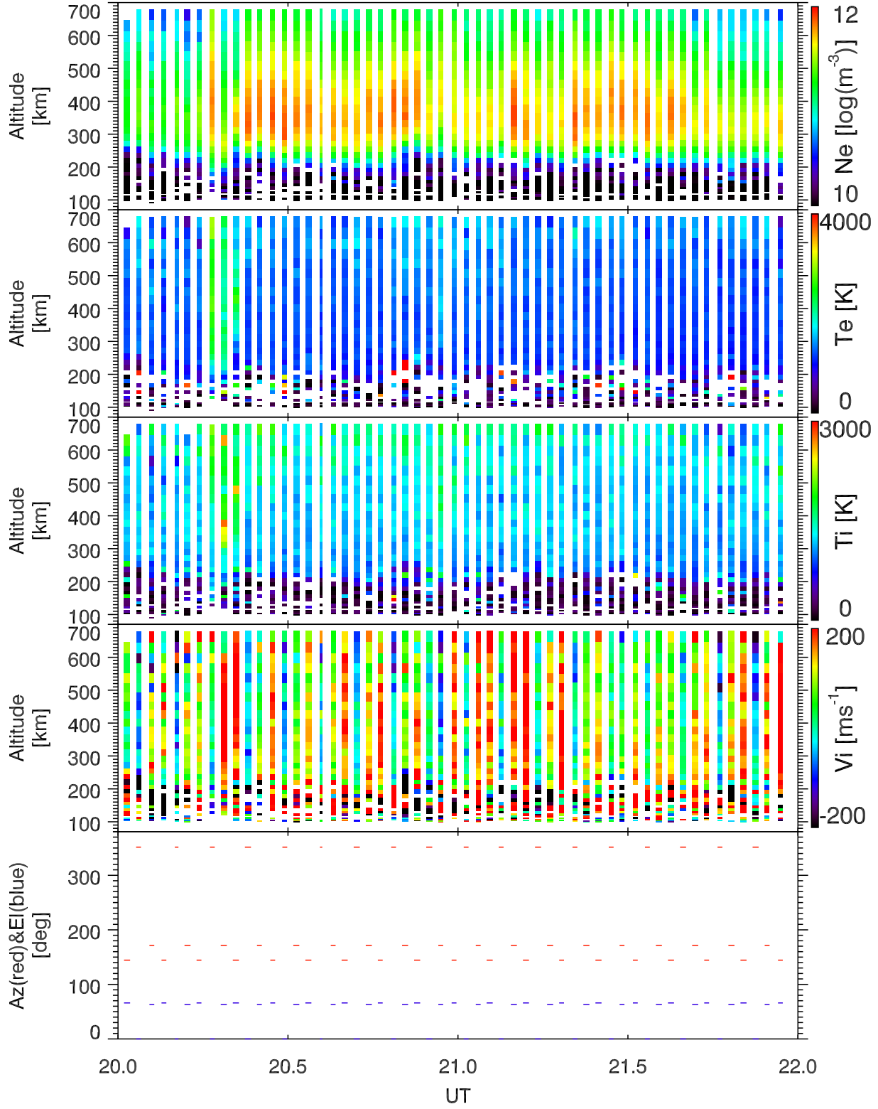
EISCAT 2001-02-20_20_22UT_tau0_ant@32m.
