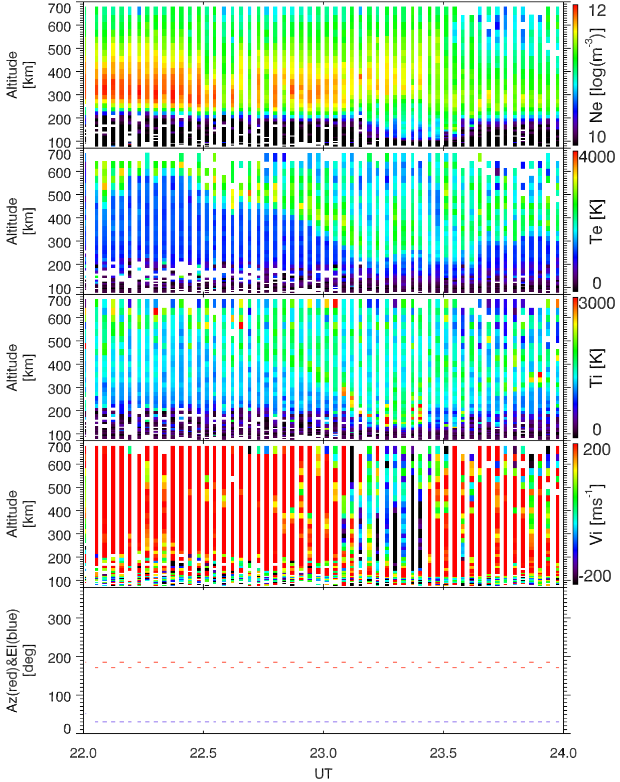
EISCAT 2001-02-20_22_24UT_tau0_ant@32m.
