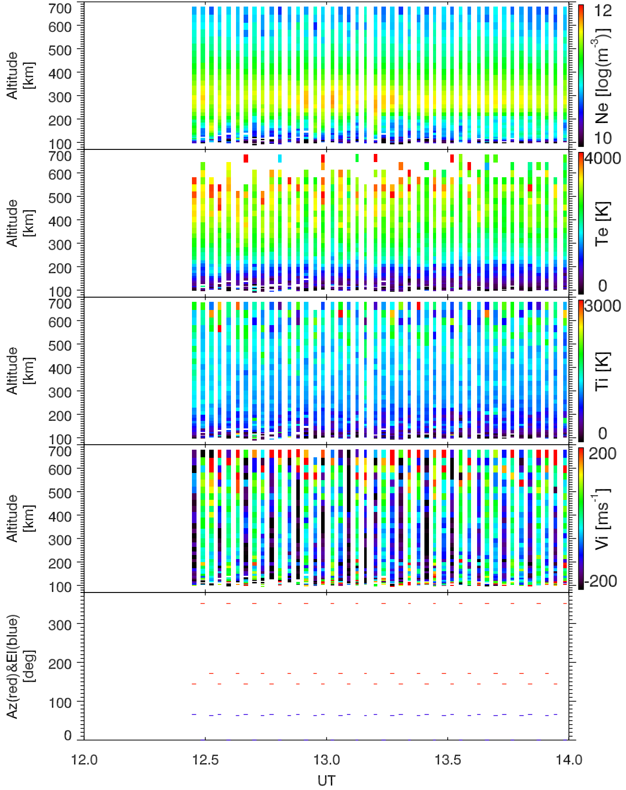
EISCAT 2001-02-21_12_14UT_tau0_ant@32m.
