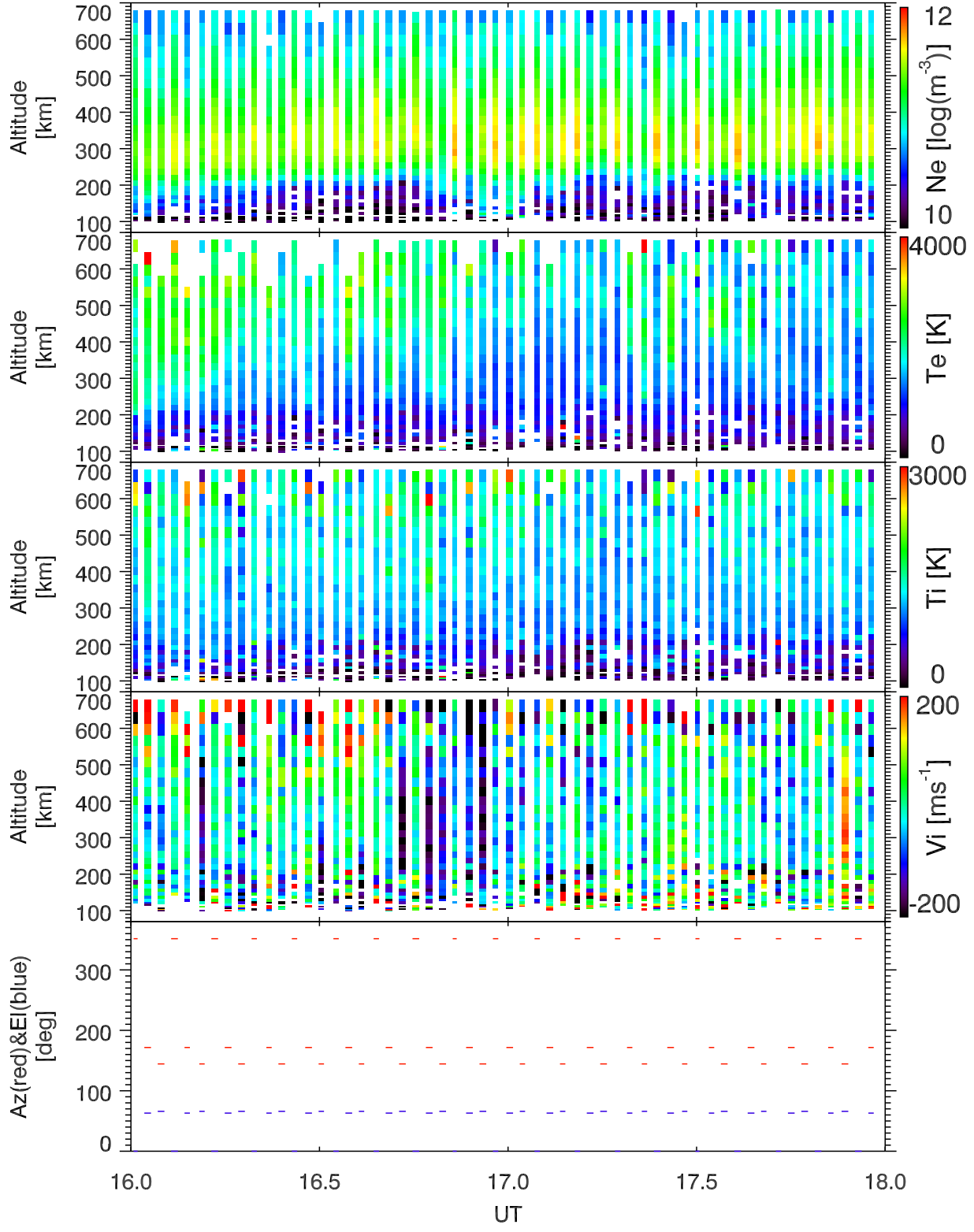
EISCAT 2001-02-21_16_18UT_tau0_ant@32m.
