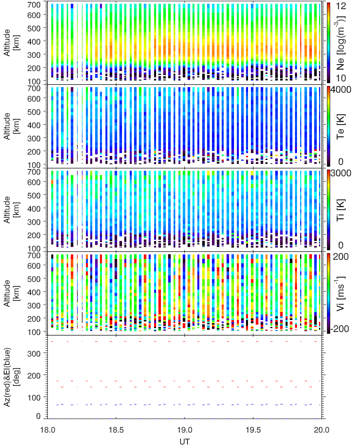
EISCAT 2001-02-21_18_20UT_tau0_ant@32m.
