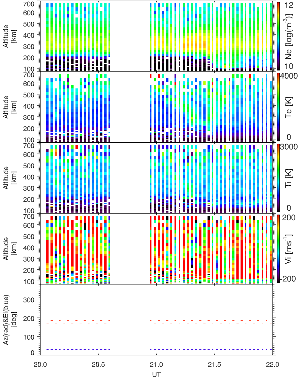
EISCAT 2001-02-21_20_22UT_tau0_ant@32m.
