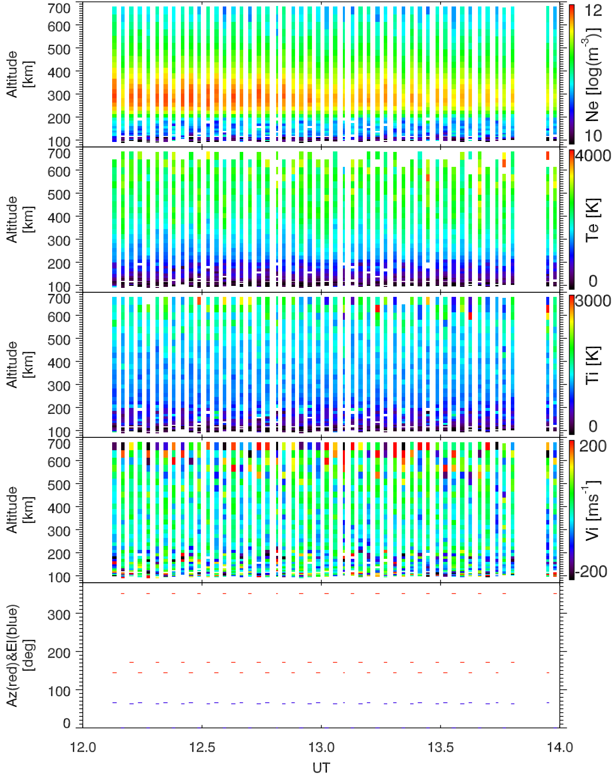
EISCAT 2001-02-22_12_14UT_tau0_ant@32m.
