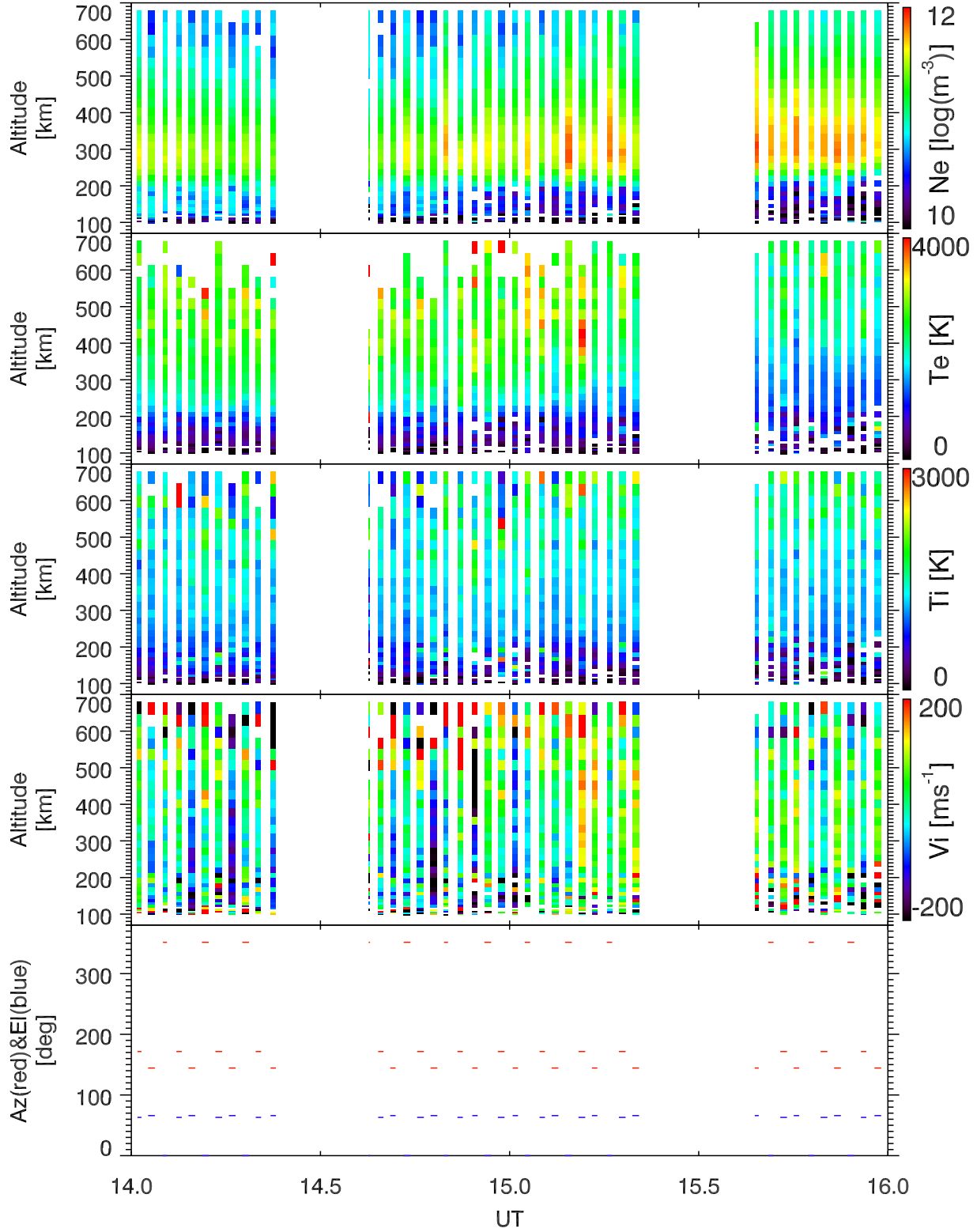
EISCAT 2001-02-22_14_16UT_tau0_ant@32m.
