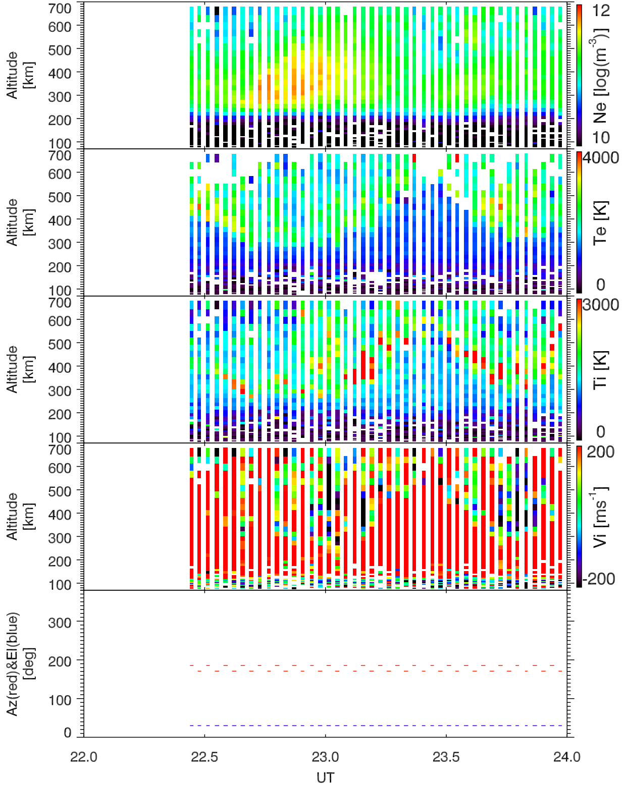
EISCAT 2001-02-22_22_24UT_tau0_ant@32m.
