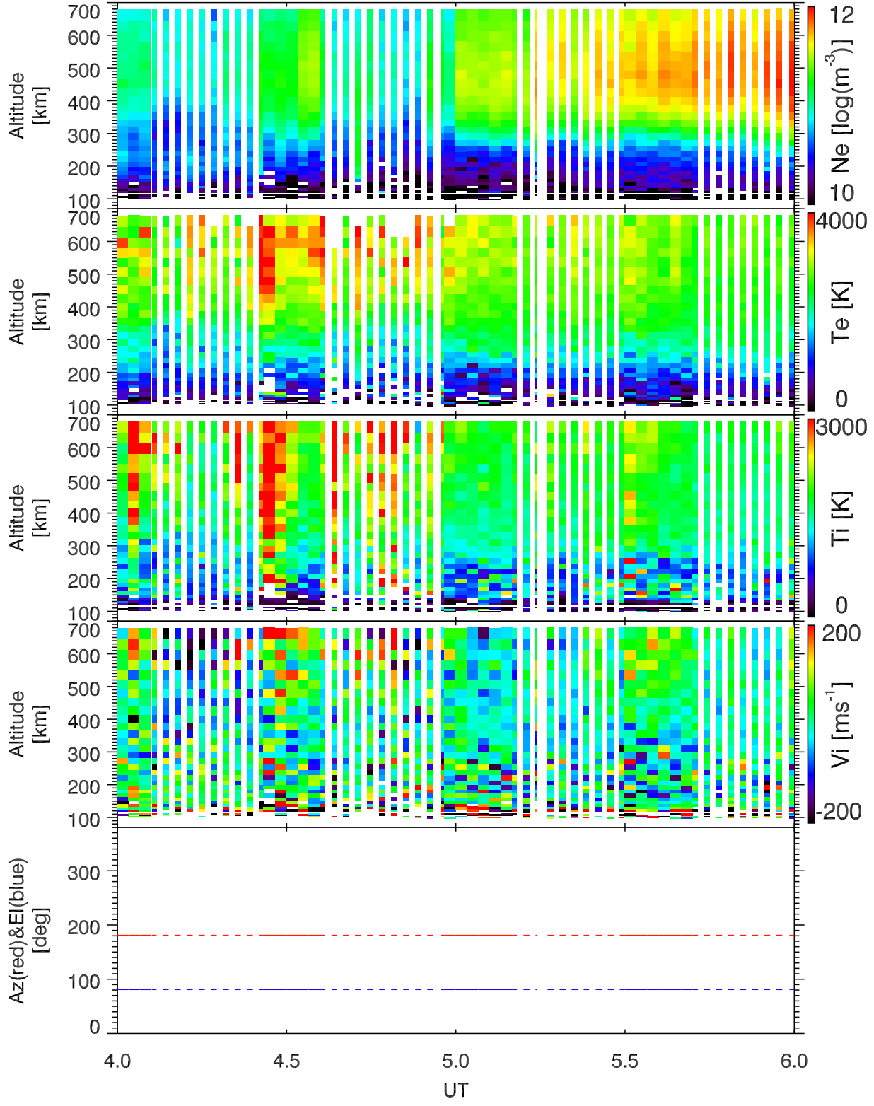
EISCAT 2001-10-20_04_06UT_tau0_120@42m.
