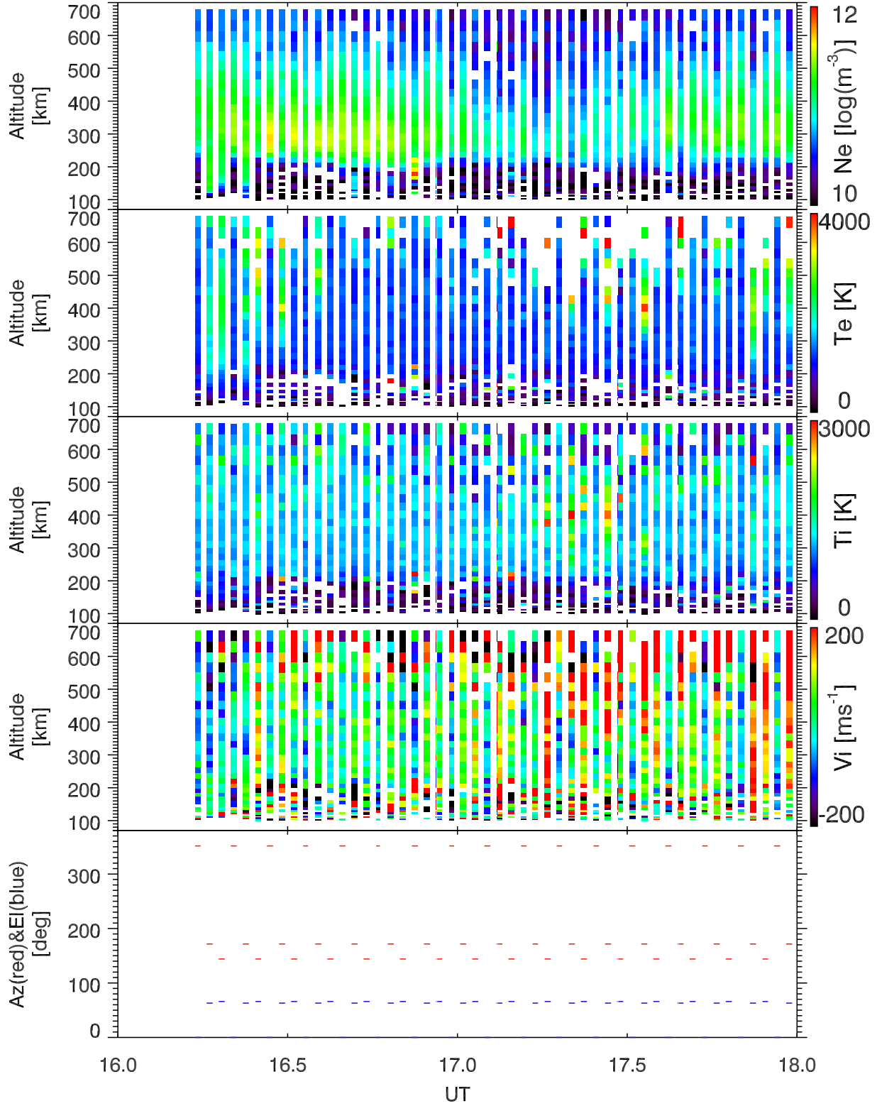
EISCAT 2001-12-11_16_18UT_tau0_ant@32m.
