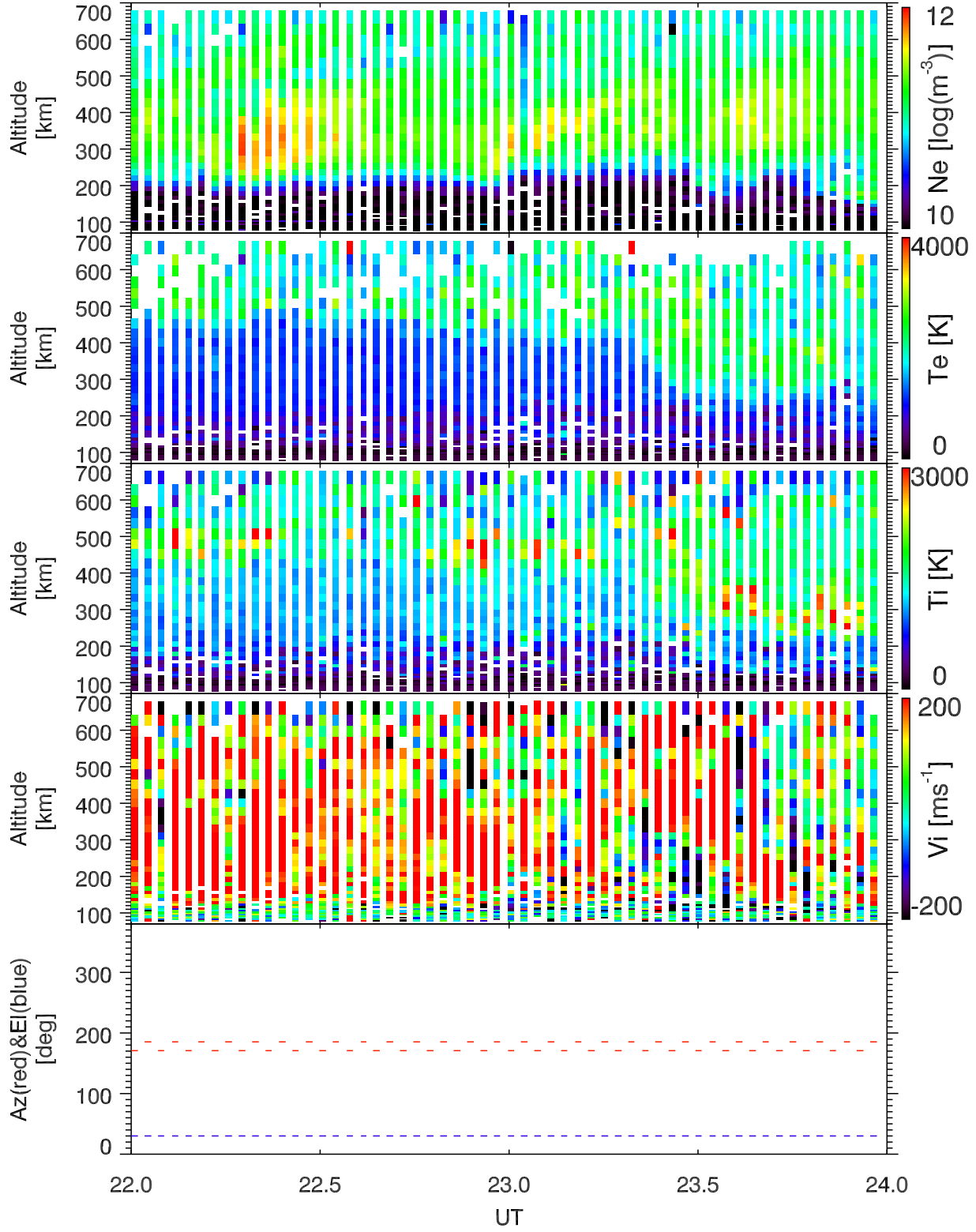
EISCAT 2001-12-11_22_24UT_tau0_ant@32m.
