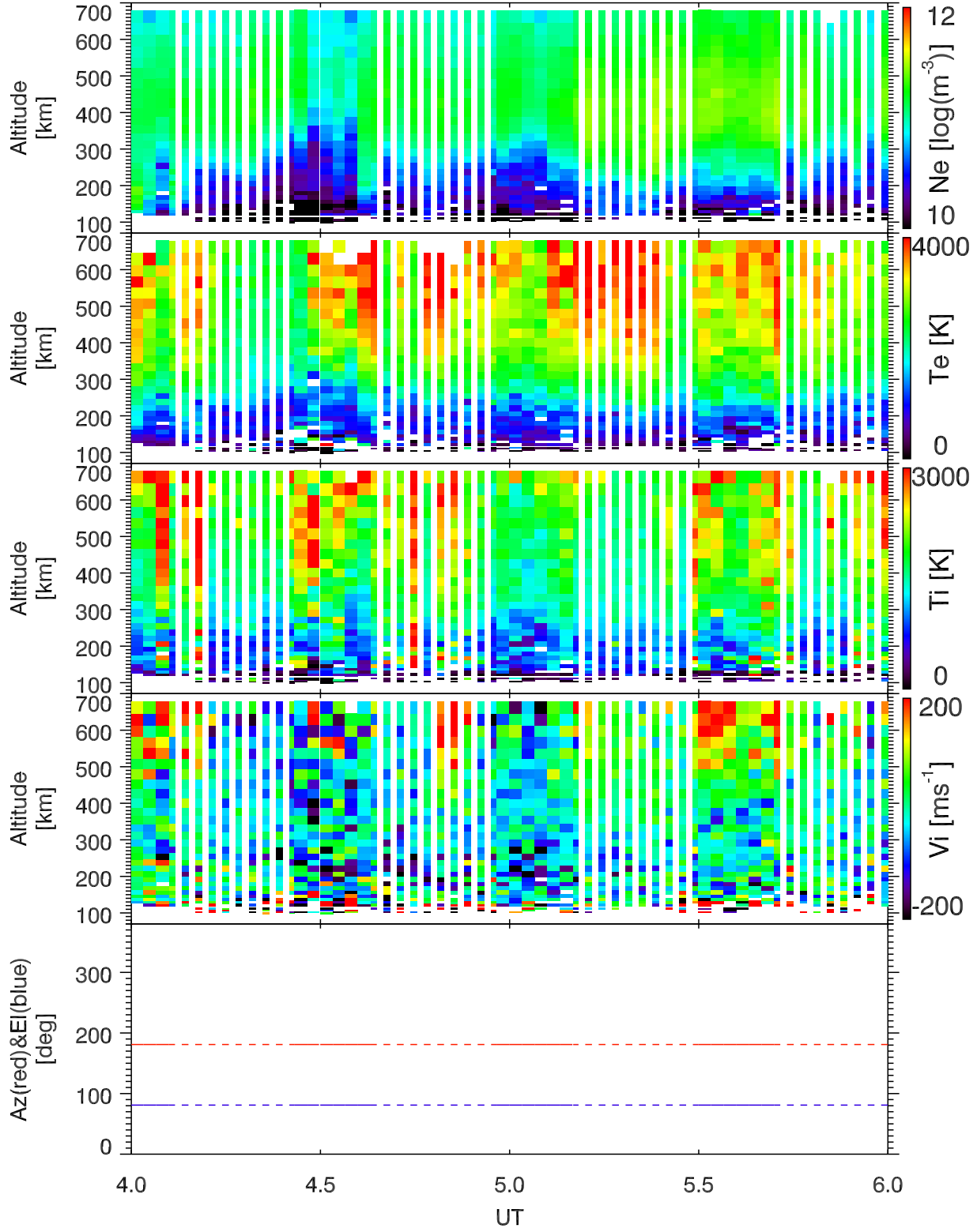
EISCAT 2001-12-12_04_06UT_tau0_120@42m.
