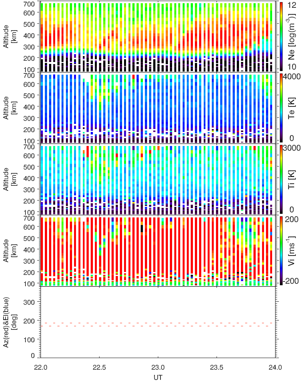
EISCAT 2001-12-12_22_24UT_tau0_ant@32m.
