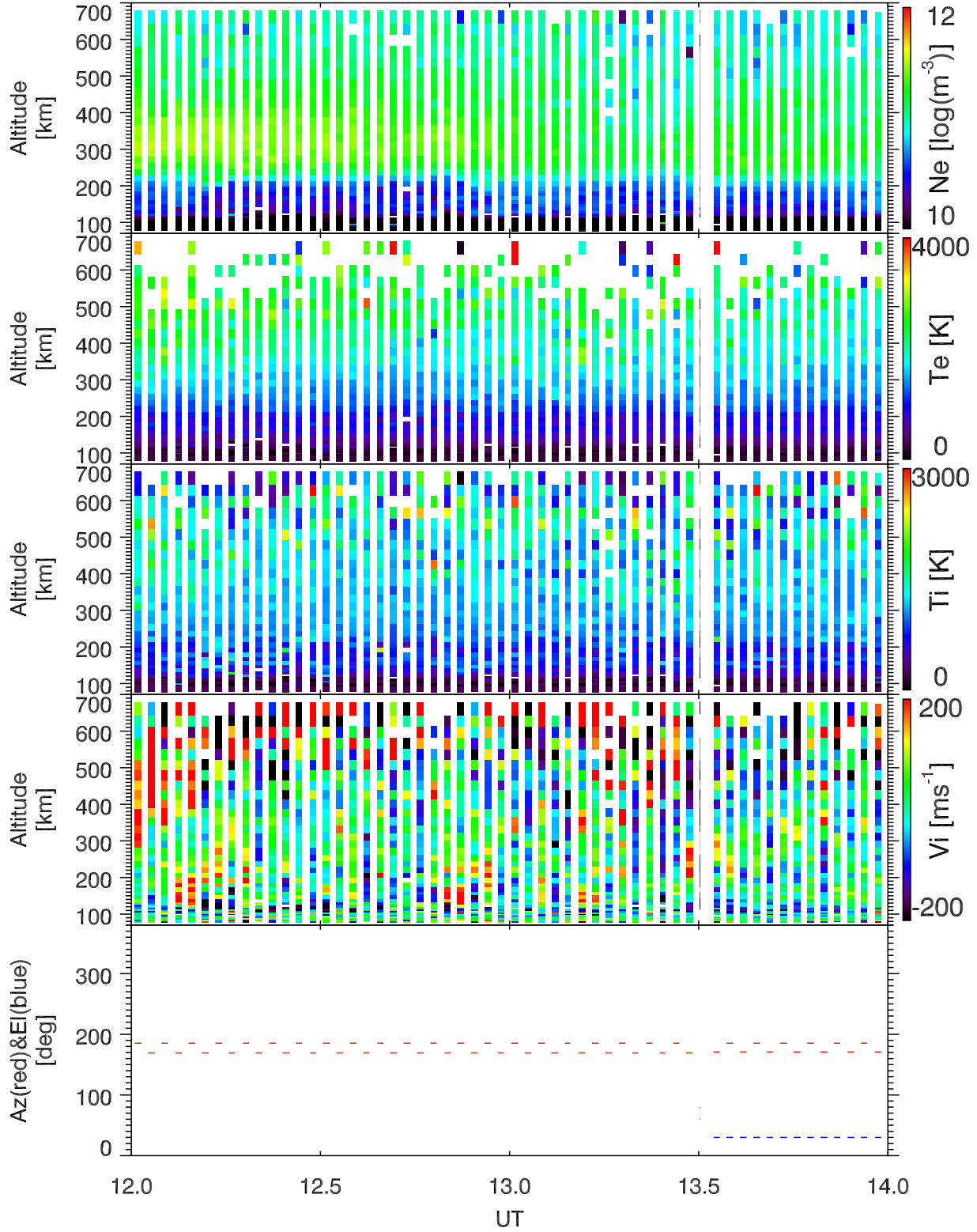
EISCAT 2001-12-13_12_14UT_tau0_ant@32m.
