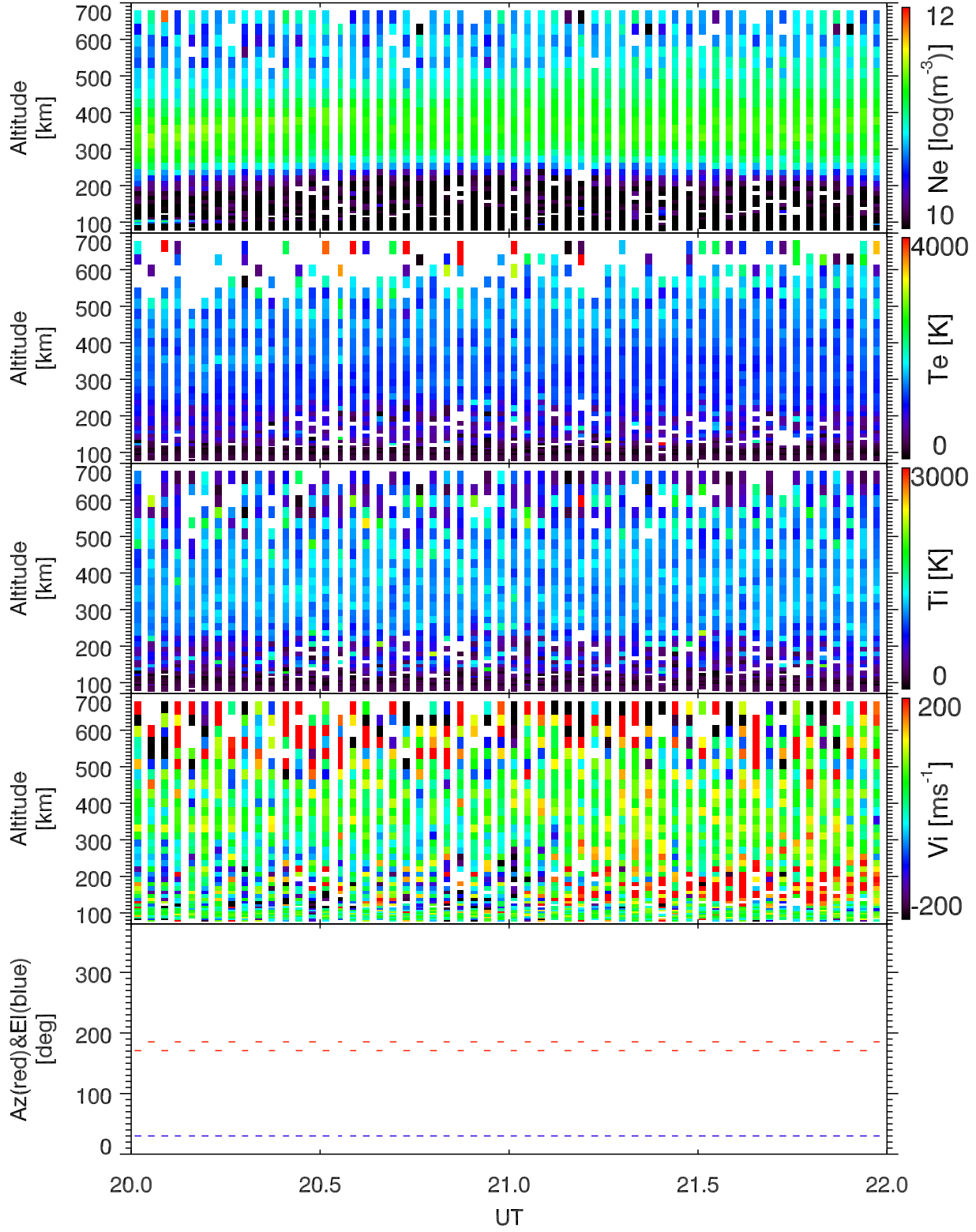
EISCAT 2001-12-13_20_22UT_tau0_ant@32m.
