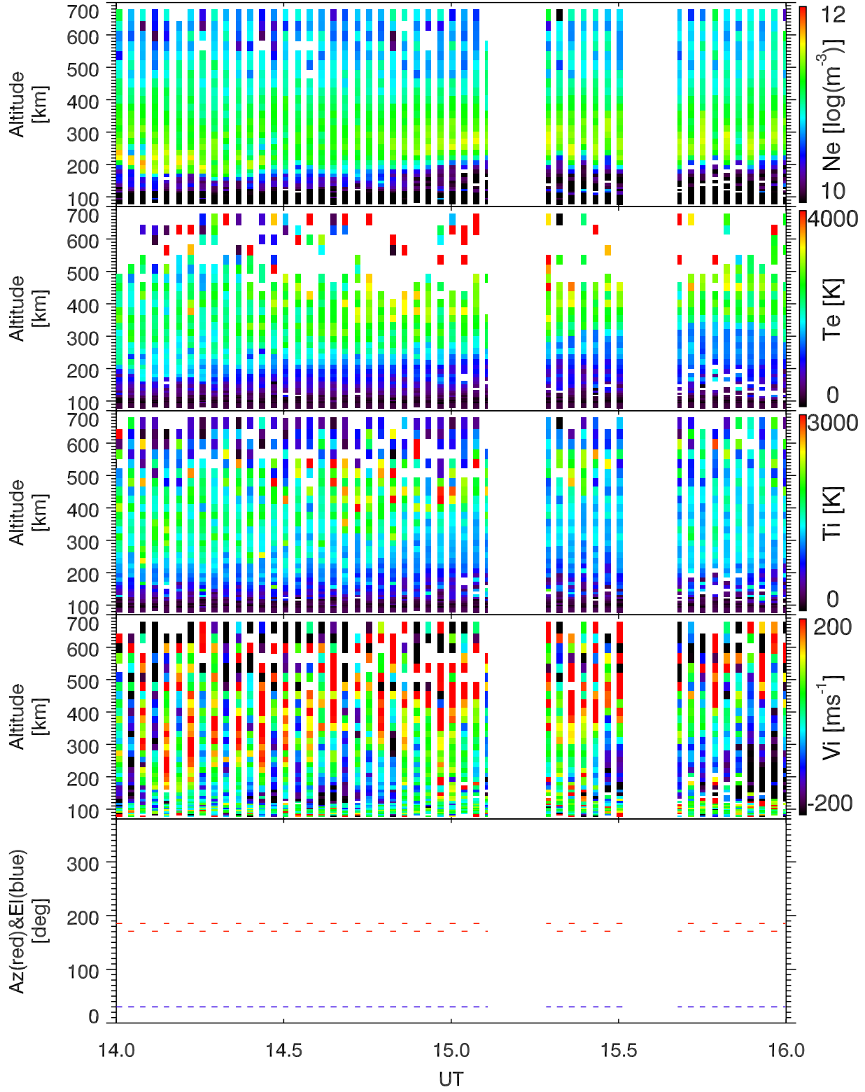
EISCAT 2001-12-14_14_16UT_tau0_ant@32m.
